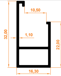
8-10 mm Cam Altı Profil 8-10 mm Glass Bottom
