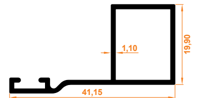
İç Açılır Fitilli Sineklik Profili Inward Foldable Flyscreen Profile
