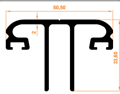
Cam Çıta Profili Glass Strip Profile
