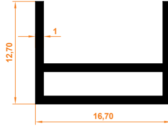
Nobel Eşiksiz Kasa Profili Nobel Case Profile without Threshold
