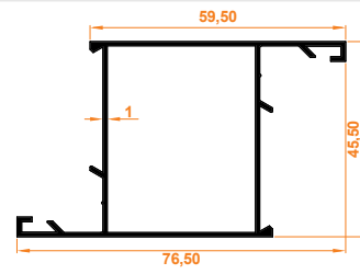
Aldoks (Orta) Kanat Profili Aldoks (Mid) Wing Profile
