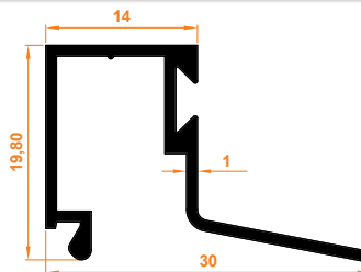
Aldoks Isıcam Çita Aldoks Double Glazing Stave
