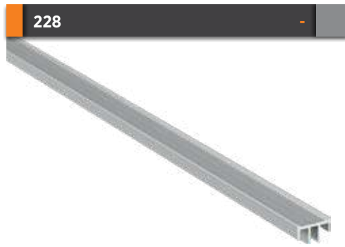
İspanyolet Karşılık Profili Espagnolette Provision Profile Paket İçi Adet Quantity Per Package 10 Gramajı Weight 0,156 kg/m
