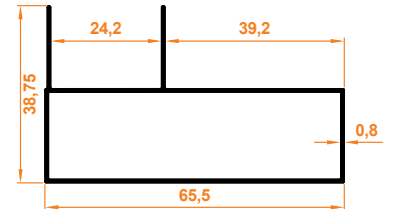
Junior Büyük Kasa Profili Junior Big Case Profile
