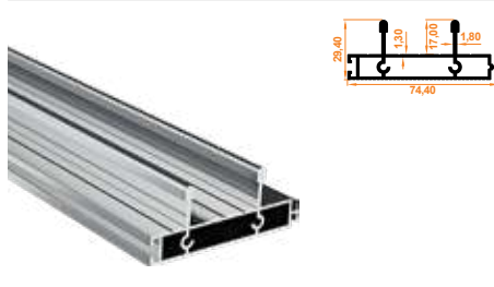
213 İkili Eşikli Alt Kasa Profil Double Threshold Lower Case Profile
