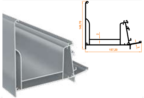
422 Oluk Profili Groove Profile
