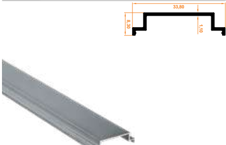
166 Açılımlı için Ray Kapatma 'L' Profil Rail Closure 'L' Profile for Opening
