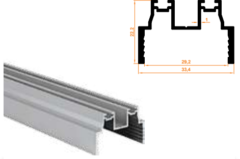
802 Düz Kapak Menteşe Profil Flat Cover Hinge Profile
