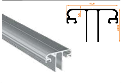
429 Cam Çitası Profili Glass Strip Profile
