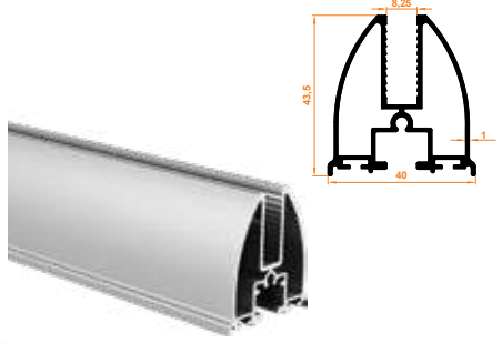
105 Fırtına Baza Profil Firtina Base Profile
