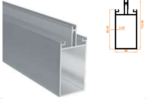
419 Orta Kayıt Profili Center Mullion Profile
