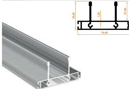
229 İkili Üst Kasa Profil Double Upper Case Profile
