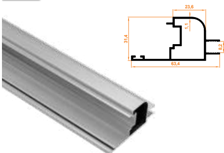
135 8 mm İspanyolet Profil 8 mm Espagnolette Profile
