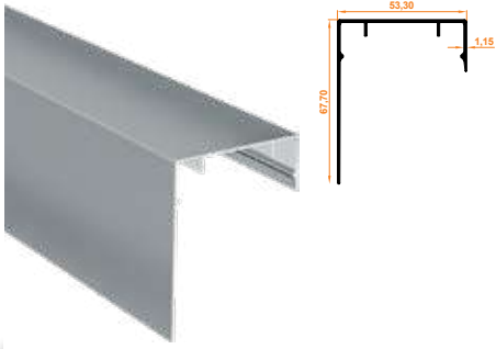
417 Sonlandırıcı Cam Çita Kapak Profili End Cap Glass Strip Cover Profile
