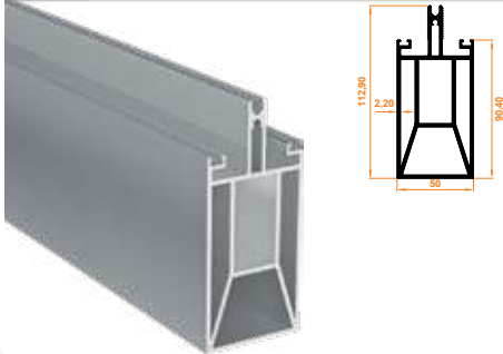
423 Destekli Orta Kayıt Profili Reinforced Center Mullion Profile
