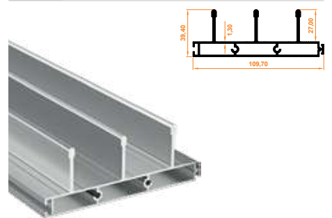
230 Üçlü Üst Kasa Profil Triple Upper Case Profile
