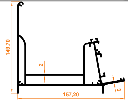
Oluk Profili Rinnenprofil
