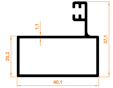
Geniş Yan Dikme Rahmenprofil (breit)
