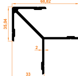
Aldoks (Orta) Köşe Takoðu Aldoks (Mid) Corner Wedge
