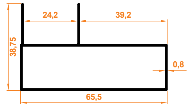
Junior Büyük Kasa Profili Junior großem Rahmenprofil
