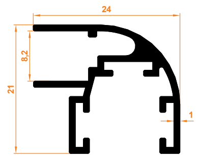
Köşe Dönüş Fitol Dichtungsprofil Eck-Rücklauf
