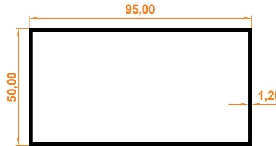
95x50 Kutu Profil 95x50 Box Profile
