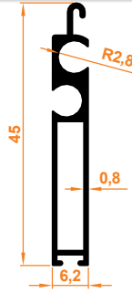
39x55 Alt Parça Kilitli Profil 39x55 Unteres Verriegelungsprofil
