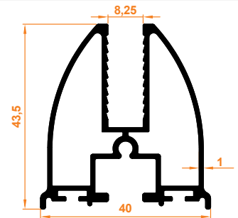
Firtına Baza Profil Firtına Bodenprofil
