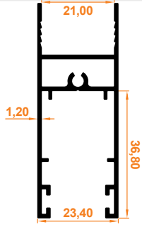
Sürme Baza Profil Schiebesystem Bodenprofil
