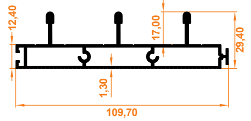
Üçlü Eşikli Alt Kasa Profil Schiene Unten mit Schwelle (dreifach)
