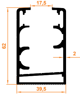
Düz Kasa Profil Flachprofil
