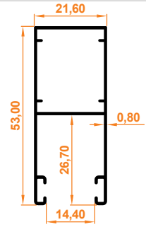
39'lik Yan Dikme 39 Side Column
