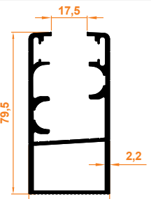
Büyük Düz Kasa Profili Großes Flachprofil
