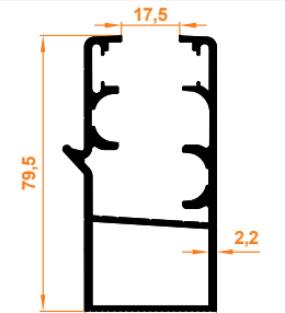
Oluklu Büyük Kasa Profili Großes Rinnenprofil
