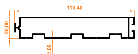
Üçlü Yan Kasa Profil Rahmenprofil (dreifach)
