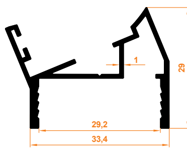
22,5° Dönüş Profil 22,5°- Drehungsprofil
