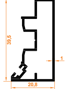
Yan Dikme Profili Rahmenprofil Isolierglas
