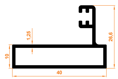
Dar Yan Dikme Rahmenprofil (schmal)
