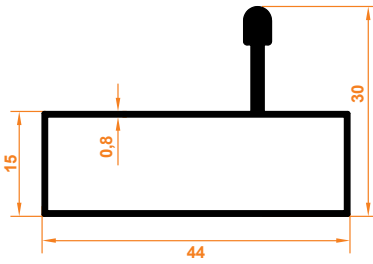
Platin Tekli Kasa Profil
