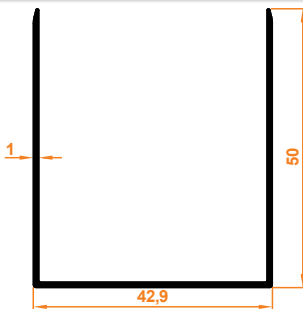
U Kapatma Profil U-Abschlussprofil
