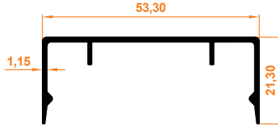
Cam Çıta Kapak Profili Glasleisten Abdeckungsprofil
