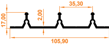
Üçlü Eşiksiz Alt Kasa Profil Schiene Unten mit niedriger Schwelle (dreifach)
