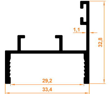
Sabit Cam İspanyolet Karşılık Profil Gegenstück Profil 8 mm Drehstangengriff für Festglas
