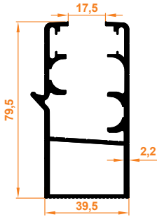
Oluklu Büyük Kasa Profil Großes Rinnenprofil
