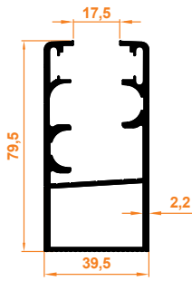
Büyük Düz Kasa Profil Großes Flachprofil
