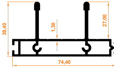
İkili Üst Kasa Profil Schieneprofil Oben (zweifach)
