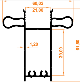
Çekme Kol Profil Griffprofil
