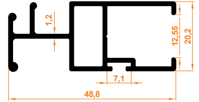
Platin Kanat Profil
