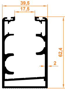
Düz Kasa Üstten Fitilli Profil Flachprofil mit Dichtung Oben
