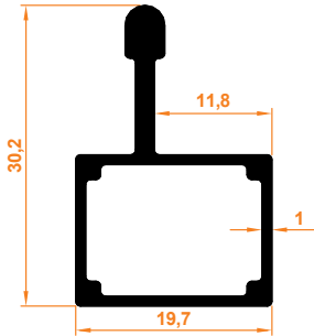
Platin Tekli Dar Kasa Profil
