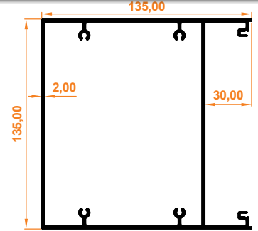
Gizli Ayak Profili Versteckter Aluminium Pfosten
