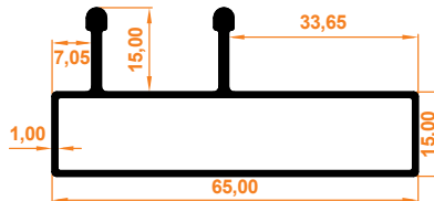
Platin Geniş Çiftli Kasa Profil
