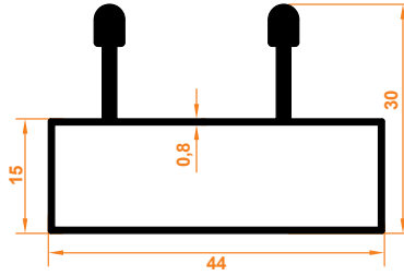
Platin Çiftli Kasa Profil
