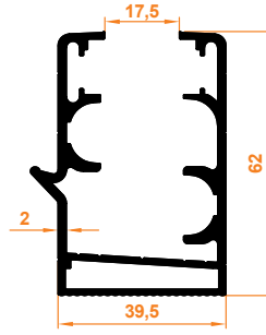
Oluklu Kasa Profil Rinnenprofil
