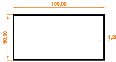
50x100 Kutu Profil 50x100 Box Profile
