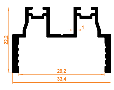
Düz Kapak Menteşe Profili Abdeckung Isolierglas-Scharnierprofil
