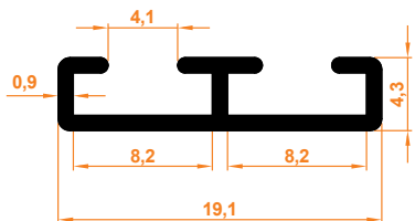
Zebra Üst Çıta Profil Zebra Oberleistenprofil
