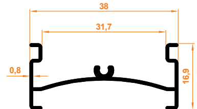
Dar Kasa Stor Profil Schmaler Kasten-Rollo-Profil
