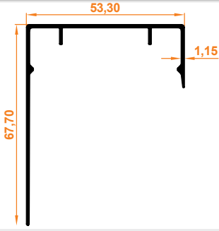
Sonlandırıcı Cam Çıta Kapak Profili Endkappe Glasleiste Abdeckprofil
