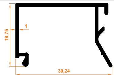
Aldoks Tek Cam Çıta Aldoks Single Glass Stave
