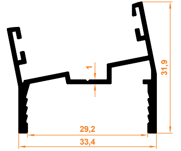
11° Dönüş Profil 11°- Drehungsprofil
