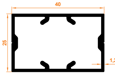
40x25 Dikme 40x25 Column
