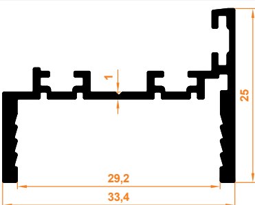
Sabit Cam Mantar Profil Scharnierprofil für Festglas
