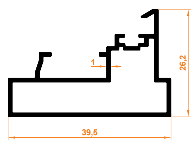
Açılır Dikme Profil Rahmenprofil Öffnend
