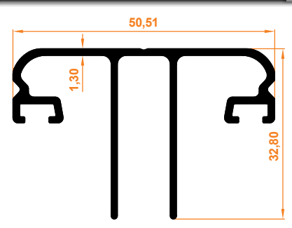
Cam Çıta Profili Glasleistenprofil
