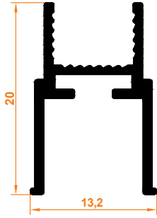
Orta H Fitol Dichtungsprofil H (mitte)
