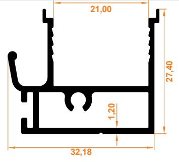
Kenet Profil Klemmprofil
