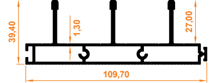
İkili Üçlü Kasa Profil Schieneprofil Oben (dreifach)
