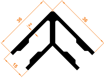
Aldoks (Dar) Köşe Takoðu Aldoks (Tight) Corner Wedge
