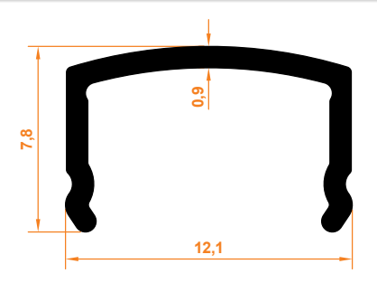
Boru Çıtası Pipe Lath
