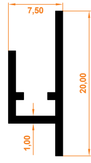
Yaylı Yapışkan Profil Spring Adhesive Profile
