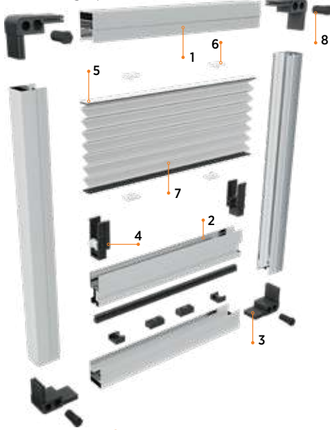
Köşeden Gergi Set İçeriği / Set-Inhalt mit Eckspann
