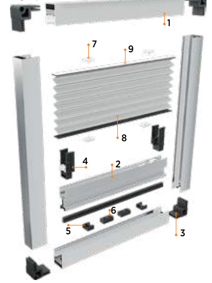
İçten Gergi Set İçeriği / Set-Inhalt mit Innenspann
