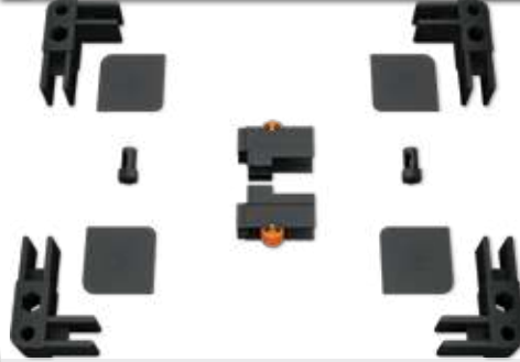
Süper Seri Köşeden Gergi Aksesuar Seti Super Serie Zubehörsatz - mit Eckspann
