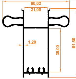
Çekme Koll Profil Pull Handle Profile
