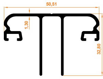
Cam Çıta Profili Glass Strip Profile
