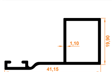
İçe Açılır Fitilli Sineklik Profili Inward Foldable Flyscreen Profile
