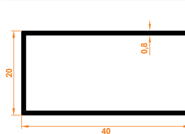
20x40 Sineklik 20x40 Fly Screen
