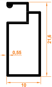
10x20 Sineklik 10x20 Fly Screen
