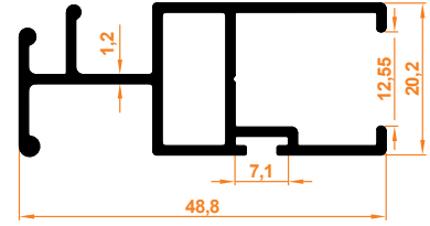
Platin Kanat Profil Platin Serie Flügelprofil
