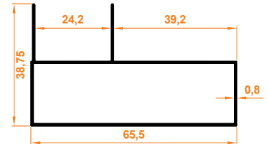
Junior Büyük Kasa Profili Junior großem Rahmenprofil
