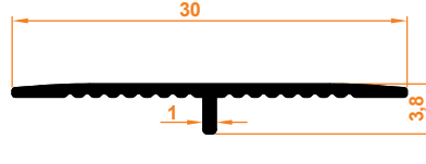
T Profili T-Verbindungsprofil
