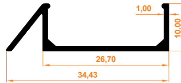
Junior Eşiksiz Kasa Profil Junior Bodenprofil - mit niedriger Schwelle
