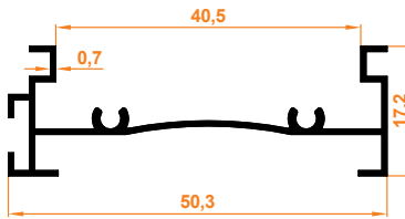
Zebra Açık Kasa Open Cassette for Zebra Blinds
