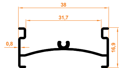
Dar Kasa Stor Profil Schmäler Kasten-Rollo-Profil
