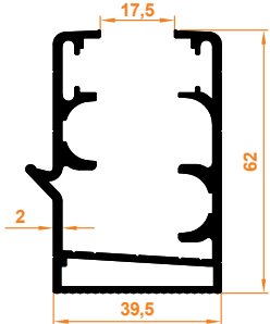
Oluklu Kasa Profili Rinnenprofil
