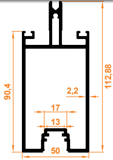
Ledli Orta Kayıt Profili Mittelprofil mit LED
