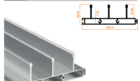
230 İkili Üçlü Kasa Profil Triple Upper Case Profile
