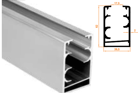
109 Düz Kasa Profil Flat Case Profile
