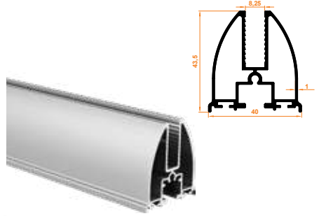
105 Fırtına Baza Profil Firtina Base Profile
