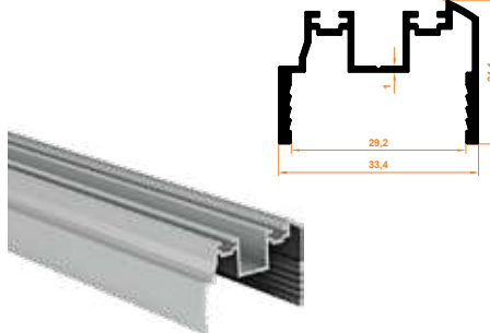
807 Açılı Dönüş Menteşe Profil PopUp Return Hinge Profile
