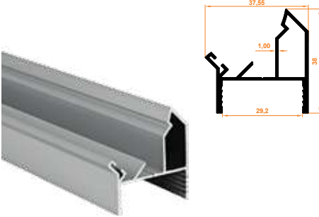
803 45° Dönüş Profil 45° Return Profile
