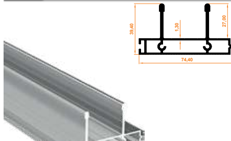
229 İkili Üst Kasa Profil Double Upper Case Profile
