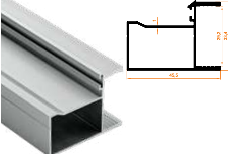
806 90° Dönüş Profil 90° Return Profile
