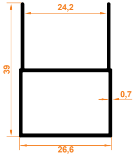
Junior Kasa Profil Junior Case Profile
