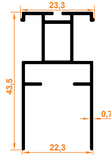
Star Kanat Profil Star Wing Profile
