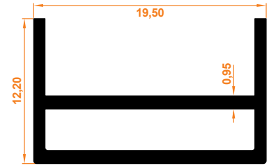
Slim Eşiksiz Profil Slim Profile without Threshold
