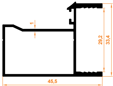
90° Dönüş Profil 90° Return Profile
