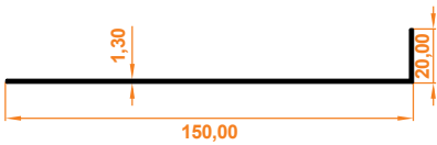
20x150 Köşebent 20x150 Angle Bracket
