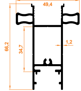
İspanyolet Çekme Kol Profili Espagnolette Pull Handle Profile
