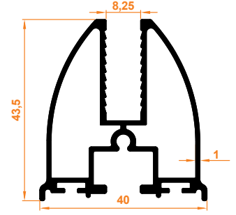
Firtina Baza Profil Firtina Base Profile
