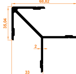
Aldoks (Orta) Köşe Takozu Aldoks (Mid) Corner Wedge
