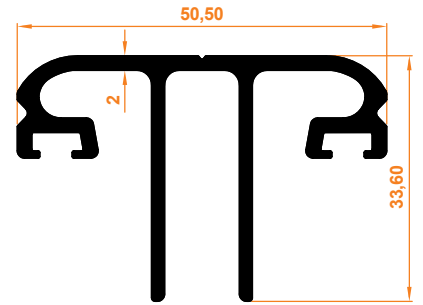
Cam Çıta Profili Glass Strip Profile
