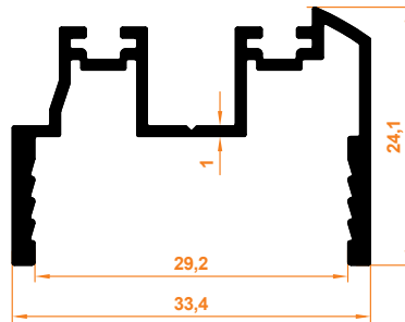
Açılı Dönüş Mentеше Profil PopUp Return Hinge Profile
