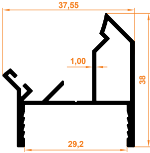
45° Dönüş Profil 45° Return Profile
