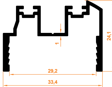
Açılı Dönüş Mentşe Profil PopUp Return Hinge Profile
