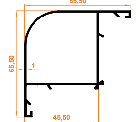
Aldoks Oval Köşe Dönüş Profili Aldoks Oval Corner Profile
