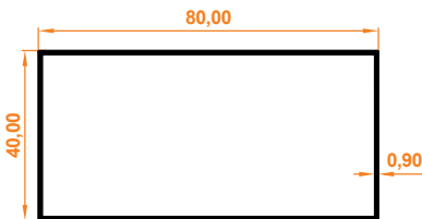
40x80 Kutu Profil 40x80 Box Profile
