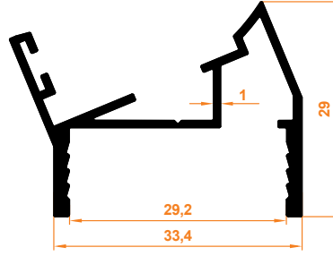
22,5° Dönüş Profil 22,5° Return Profile
