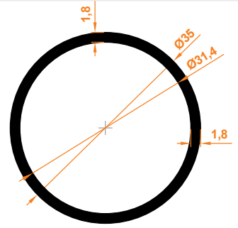
35x1,8 Boru 35x1,8 Pipe
