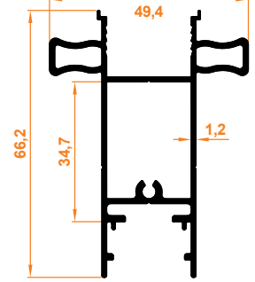
İspanyolet Çekme Koll Profili Espagnolette Pull Handle Profile
