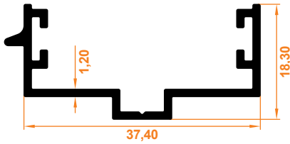
Birleřtirme Karřılık Profil Combination Provisions Profile
