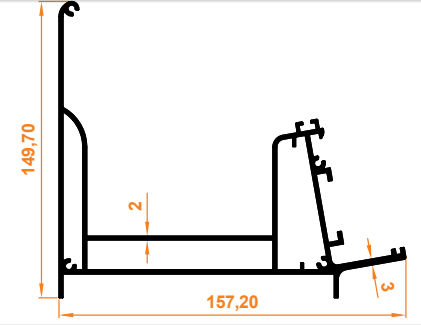
Oluk Profili Groove Profile
