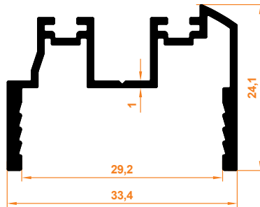
Açılı Dönüş Mantese Profili PopUp Return Hinge Profile
