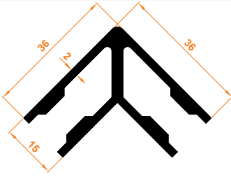
Aldoks (Dar) Köşe Takozu Aldoks (Tight) Corner Wedge
