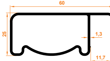
60x25 Yandan Kanallı 60x25 Side Slot
