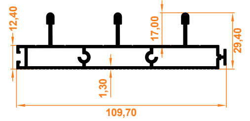
Üçlü Eřikli Alt Kasa Profil Triple Threshold Lower Case Profile
