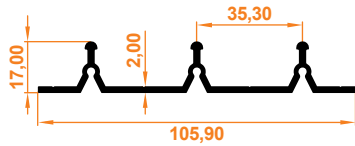
Üçlü Eřiksiz Alt Kasa Profil Triple Bottom Case Profile without Threshold
