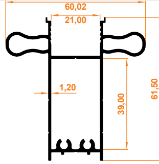
Çekme Køl Profil Pull Handle Profile
