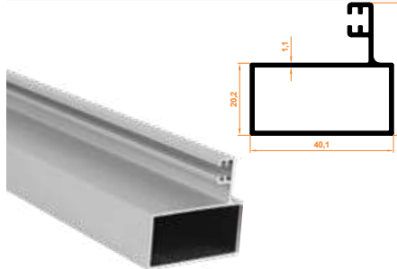
108 Geniş Yan Dikme Profil Rahmenprofil (breit)
