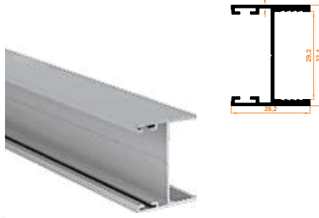
801 Düz Kapak Profil Isolierglas-Flachabdeckprofil
