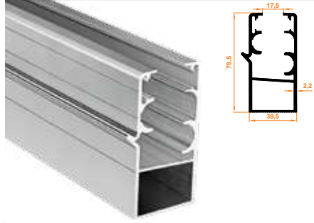
106 Oluklu Büyük Kasa Profil Großes Rinnenprofil
