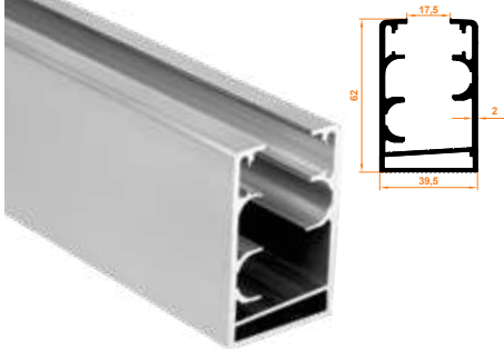
109 Düz Kasa Profil Flachprofil
