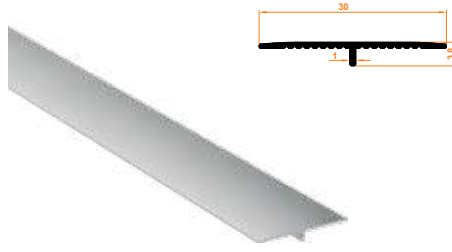
431 T Profili T-Verbindungsprofil
