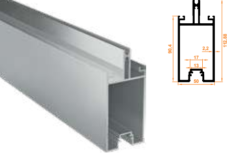
430 Ledli Orta Kayıt Profili Mittelprofil mit LED
