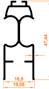
Dark Perde Kanat Profil Dark Blind Wing Profile
