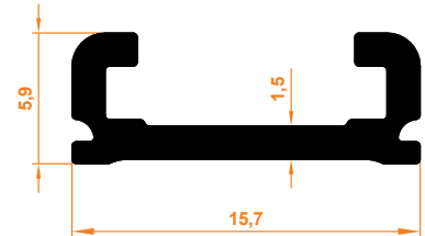
Portray Yapışkan Profil Adhesive Profile
