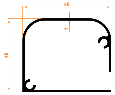
Stor Kasa Profil Stor Fallprofil
