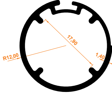
Stor Boru Profil Stor Rohrprofil
