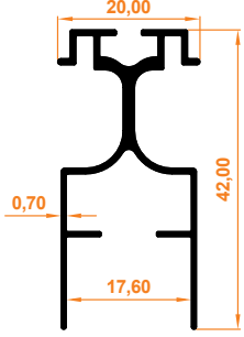
Süper Seri Kanat Profili Super Flügelprofil
