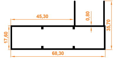
Süper Büyük Kasa Profili Super Großserie Rahmenprofil
