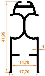
Nobel Kanat Profili Nobel Flügelprofil
