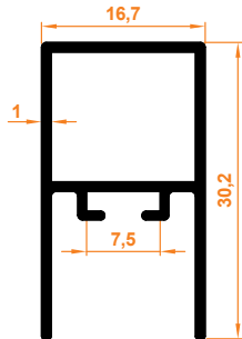
Nobel Mıknatıs Yuvalı Kasa Profili Nobel Magnetkanal-Rahmenprofil
