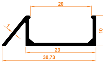
Süper Eşiksiz Kasa Profil Super-Türrahmenprofil ohne Schwelle
