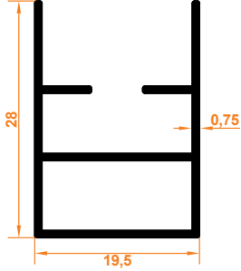
Slim Kasa Profil Slim Rahmenprofil
