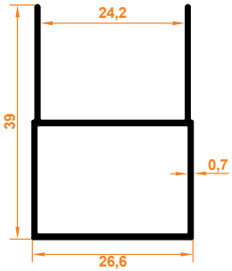
Junior Kasa Profil Junior Rahmenprofil
