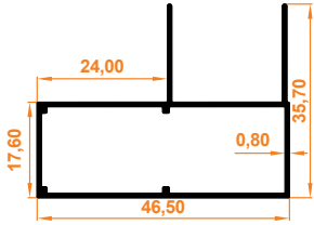
Süper Orta Kasa Profili Super-Mittelrahmenprofil
