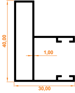
Stor Yan Kasa Profil Stor Rahmenprofil
