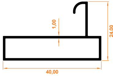
Stor Alt Kasa Profil Stor Bodenprofil
