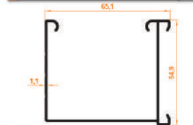
Ahşap Jaluzi Perde Kasa Profil Venetian Blind Headrail Profile Paket İçi Adet Quantity Per Package 6 Gramajı Weight 0,605 kg/m
