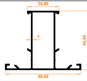
Aldoks (Dar) Orta Kayıt Profili Aldoks (Tight) Mid Entry Profile
