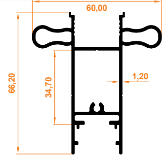
İspanyolet Çekme Kol Profili Espagnolette Pull Handle Profile
