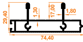
İkili Eşikli Alt Kasa Profil Double Threshold Lower Case Profile
