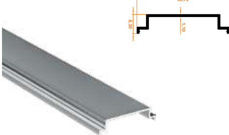
149 Açılımsız için Ray Kapatma 'L' Profil Rail Closure 'L' Profile for Non-Opening
