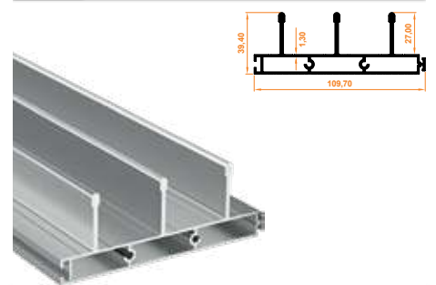
230 Üçlü Üst Kasa Profil Triple Upper Case Profile
