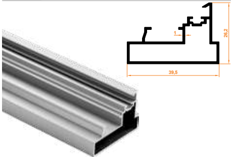
822 Açılır Dikme Profil Pop-up Column Profile
