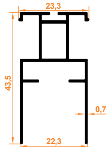
Junior Kanat Profil Junior Wing Profile
