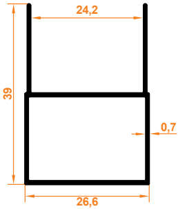
Junior Kasa Profil Junior Case Profile
