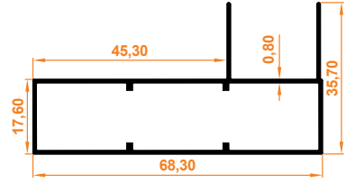
Süper Büyük Kasa Profili Super Big Case Profile
