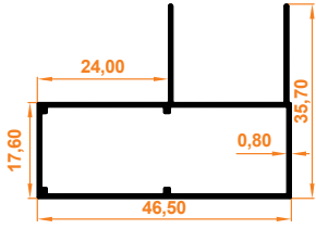
Süper Orta Kasa Profili Super Middle Case Profile
