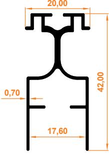
Süper Seri Kanat Profili Super Wing Profile
