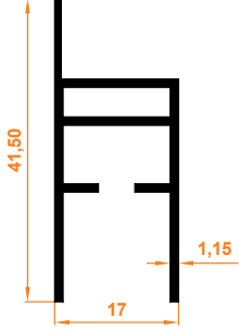
Nobel İçten Montajlı Kasa Profili Nobel Internal Mounted Case Profile
