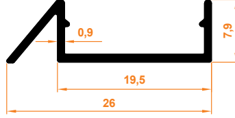
Slim Eşiksiz Profil Slim Profile without Threshold
