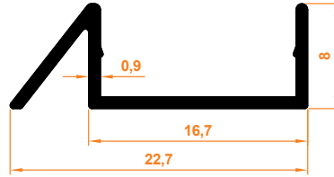
Nobel Eşiksiz Profili Nobel Profile without Threshold
