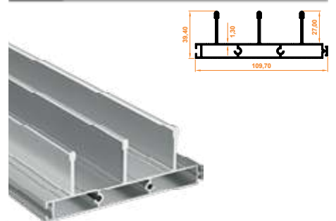
230 İkili Üçlü Kasa Profil Triple Upper Case Profile
