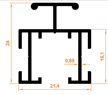
Çiftli Orta Profil Mittleres Doppelprofil
