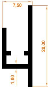
Yaylı Yapışkan Profil Kleprofil mit Spannfeder
