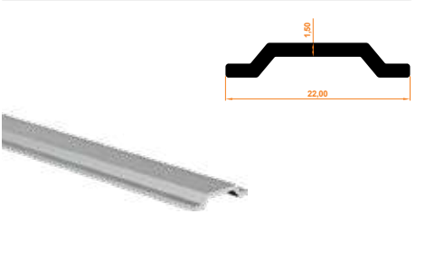
815 Tij Profil Espagnolette Profile
