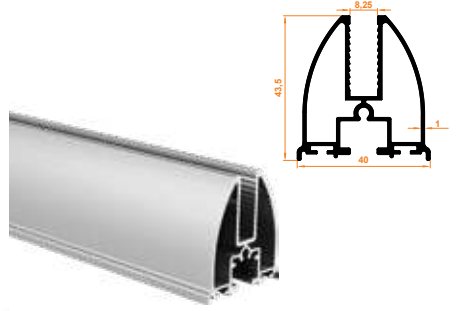
105 Fırtına Baza Profil Firtına Base Profile firtına
