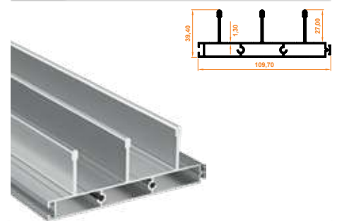
230 İkilil Üçlü Kasa Profil Triple Upper Case Profile
