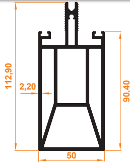
Mukavemetli Orta Kayıt Profili Reinforced Center Mullion Profile
