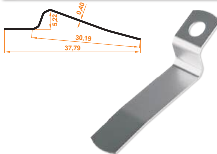
Dıştan Montajlı Metal Klips Externally Mounted Metal Clip
