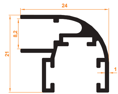
Köşe Dönüş Fitil Corner Return Wick
