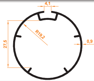
Zebra Perde Borusu Zebra Blind Tube
