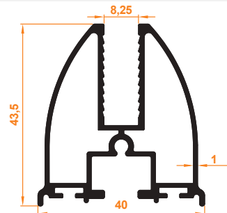
Fırtına Baza Profil Fırtına Base Profile
