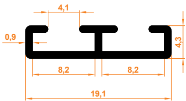
Zebra Üst Çıta Profil Zebra Oberleistenprofil
