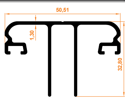
Cam Çita Profili Glasleistenprofil
