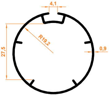
Zebra Perde Borusu Zebra Blind Tube
