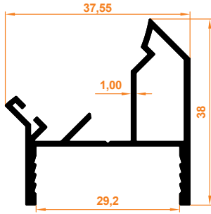
45° Dönüş Profil 45°-Drehungsprofil
