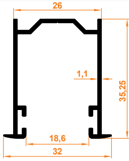
Kulaklı Kutusuz Dikme Profil Laschenbefestigtes Kastenloses Pfostenprofil
