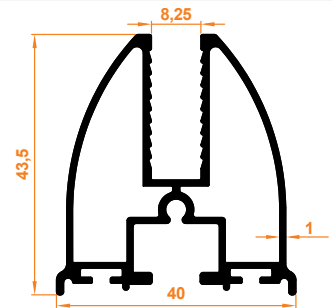
Fırtına Baza Profil Fırtına Bodenprofil
