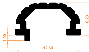
Yaylı Portray Profil Portray-Profil mit Feder
