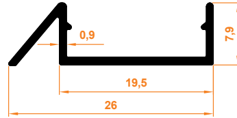
Slim Eşiksiz Profil Slim Bodenprofil - mit niedriger Schwelle
