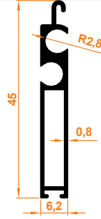
39x55 Alt Parça Kilitli Profil 39x55 Unteres Verriegelungsprofil
