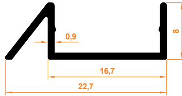
Nobel Eşiksiz Profili Nobel Bodenprofil - mit niedriger Schwelle
