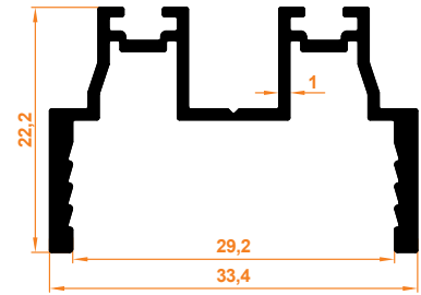
Düz Kapak Menteşe Profili Abdeckung Isolierglas-Scharnierprofil
