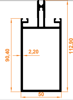
Orta Kayıt Profili Aluminium Sparren
