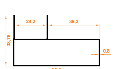
Junior Büyük Kasa Profili Junior großem Rahmenprofil
