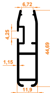
Zebra Dekoratif Lama Profil Zebra Dekorative Lamellenprofil
