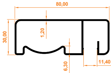
80x30 Yandan Kanallı 80x30 Side Slot
