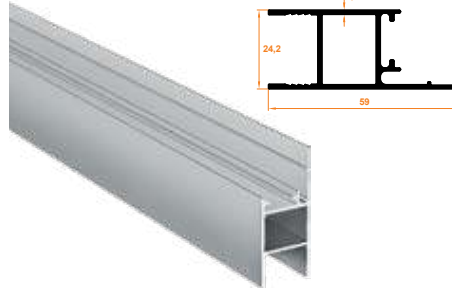
174 İspanyollet Dikme Profil Espagnolette Mullion Profile
