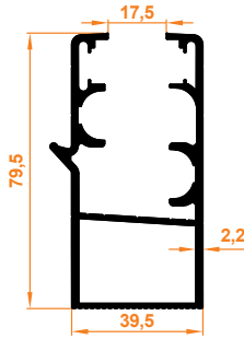
Oluklu Büyük Kasa Profil Corrugated Big Case Profile
