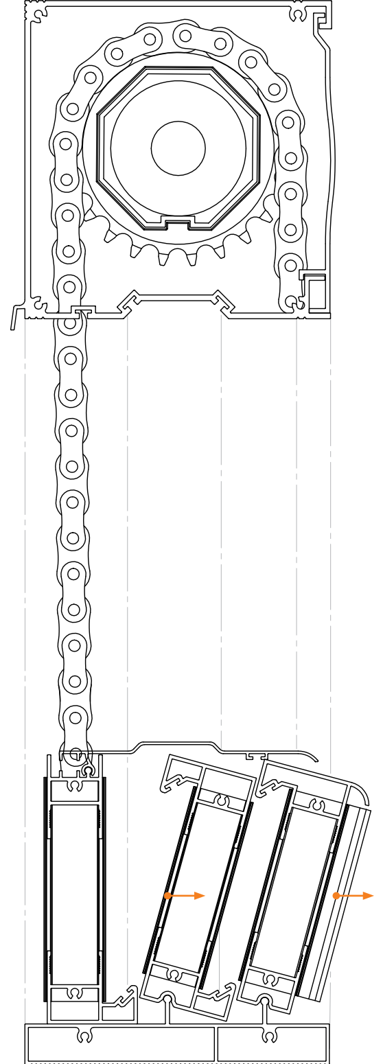
3. Kademe - Level 3
