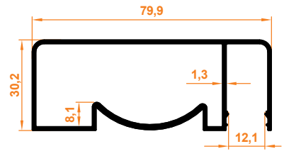
80x30 Yandan Kanallı 80x30 Side Channel
