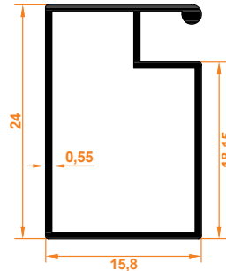
17x25 Sineklik 17x25 Fly Screen
