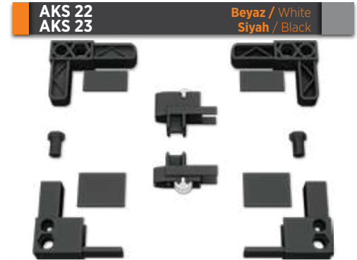
Nobel Köşeden Gergi Eşiksiz Aksesuar Seti Nobel Corner Tensioner Accessory Set without Threshold
