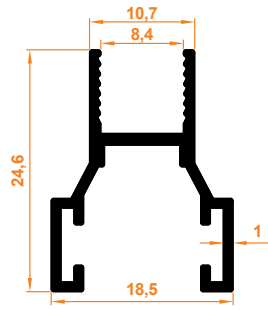
Büyük H Fitol Big H Wick
