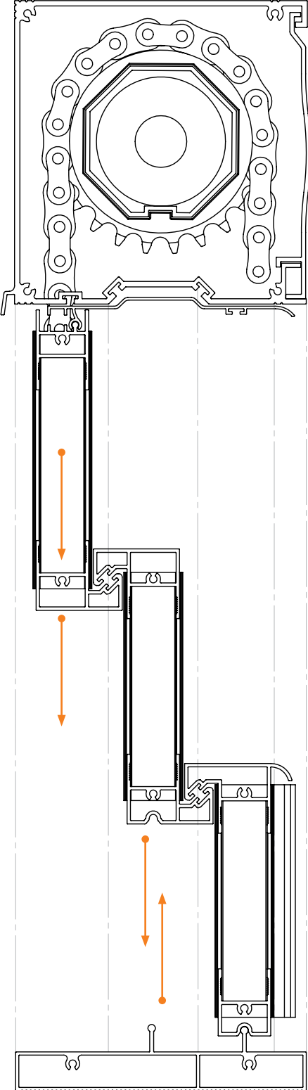
1. Kademe - Level 1
