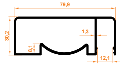
80x30 Yandan Kanallı 80x30 Side Channel
