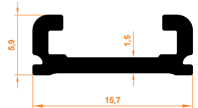
Portray Yapışkan Profil Adhesive Profile
