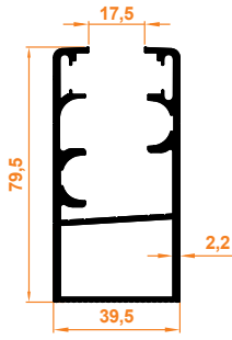
Büyük Düz Kasa Profil Big Flat Case Profile
