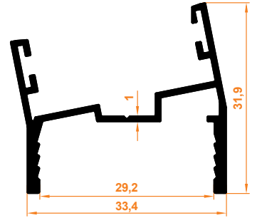
11° Dönüş Profil 11° Return Profile
