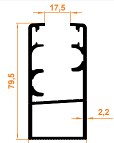
Büyük Düz Kasa Profili Big Flat Case Profile
