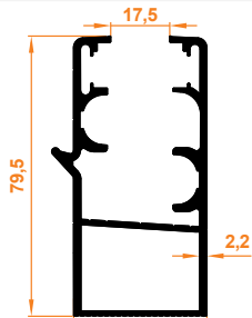
Oluklu Büyük Kasa Profili Corrugated Big Case Profile
