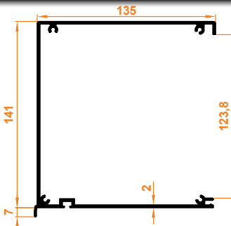
Üst Kasa Profil Top Frame Profile
