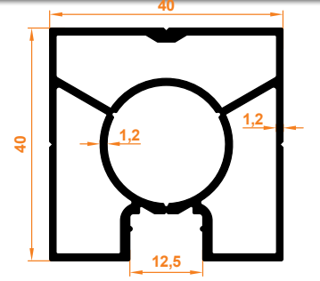
40x40 Tek Kanallı Dikme 40x40 Single Channel Column
