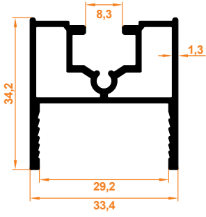
Baza Profil Base Profile
