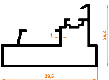
Açılır Dikme Profili PopUp Column Profile
