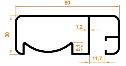
80x30 Yandan Kanallı 80x30 Side Channel
