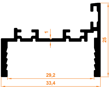
Sabit Cam Menteşe Profil Stable Glass Hinge Profile
