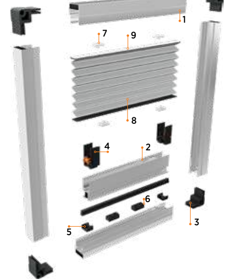
İçten Gergi Set İçeriği / Internal Tensioner Set Contents
