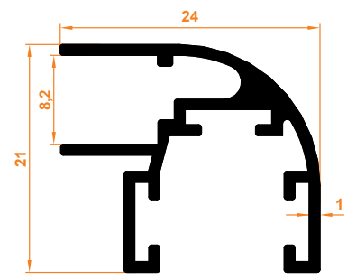
Köşe Dönüş Fitol Corner Return Wick
