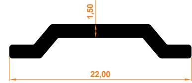
Tij Profil Espagnolette Profile
