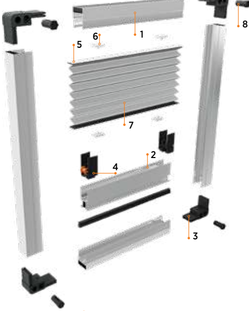
Köşeden Gergi Set İçeriği / Corner Tensioner Set Contents
