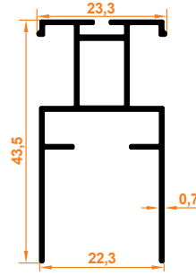
Star Kanat Profil Star Wing Profile
