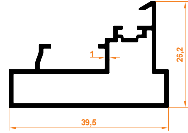
Açılır Dikme Profil PopUp Column Profile
