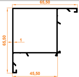
Aldoks Köşe Dönüş Profili Aldoks Corner Profile
