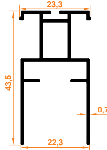
Star Kanat Profil
