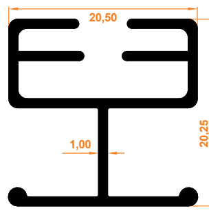
20'lik T Profil 20 T Profile
