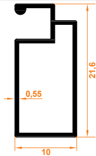
10x20 Sineklik 10x20 Fly Screen
