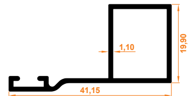
İçe Açılır Fitilli Sineklik Profili Inward Foldable Flyscreen Profile
