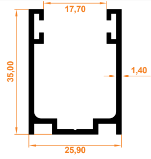
55'lik Kutusuz Dikme 55 Side Column Boxless
