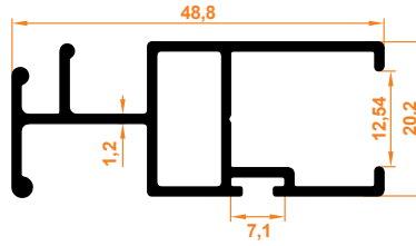
Platin Kanat Profil Platin Wing Profile
