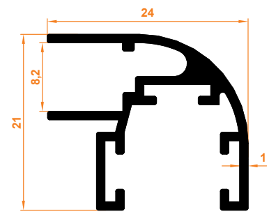
Köşe Dönüş Fitol Corner Return Wick
