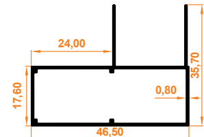
Süper Orta Kasa Profili Super Middle Case Profile
