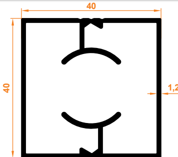
40x40 Kanalsız Dikme 40x40 Non Channel Column
