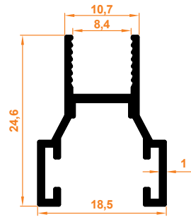
Büyük H Fitol Big H Wick
