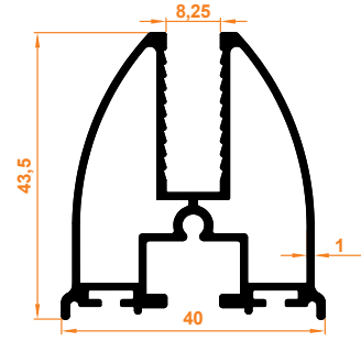
Firtına Baza Profil Firtına Base Profile
