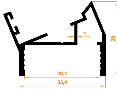
22,5° Dönüş Profili 22,5° Return Profile
