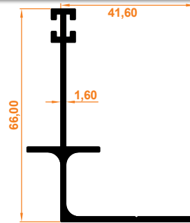
Açılımsız Çift Fitil Yan Ray L Kasa Profil Double Weatherstrips Without Opening Side L Case Profil
