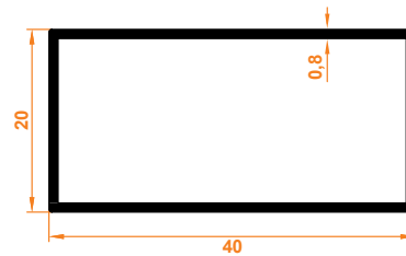
20x40 Sineklik 20x40 Fly Screen
