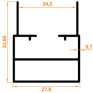
Star Kasa Profil
