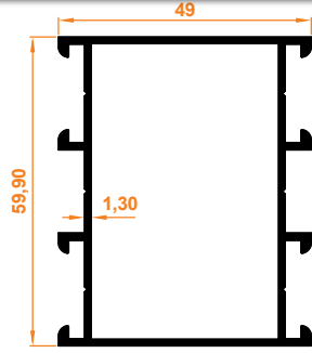
C60 Kasa Orta Kayıt Profili C60 Case Mid Entry Profile
