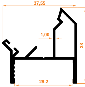
45° Dönüş Profili 45° Return Profile
