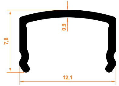
Boru Çıtası Pipe Lath
