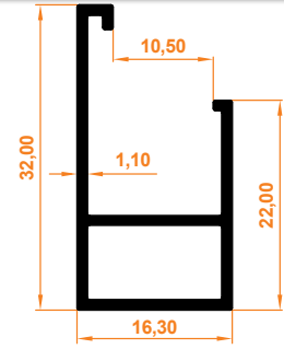
8-10 mm Cam Altı Profil 8-10 mm Glass Bottom
