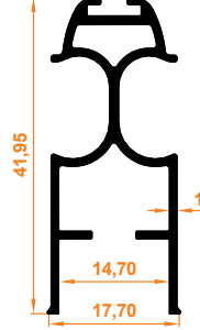
Nobel Kanat Profili Nobel Wing Profile
