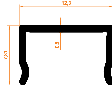
Kare Çıta Square Slot
