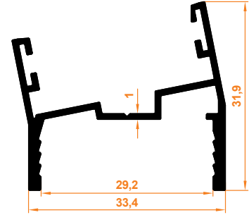
11° Dönüş Profili 11° Return Profile
