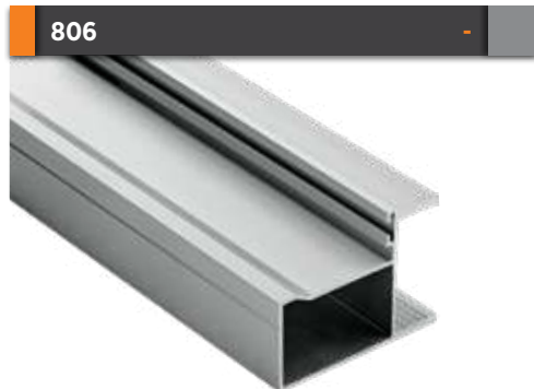
806 90° Dönüş Profil 90° Return Profile Paket İçi Adet Quantity Per Package 6 Gramajı Weight 0,475 kg/m
