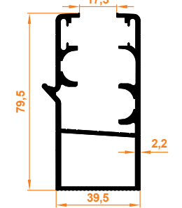
Oluklu Büyük Kasa Profili Corrugated Big Case Profile
