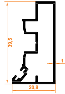
Yan Dikme Profili Side Column Profile
