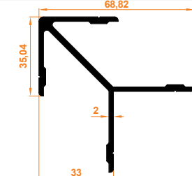
Aldoks (Orta) Köşe Takozu Aldoks (Mid) Corner Wedge
