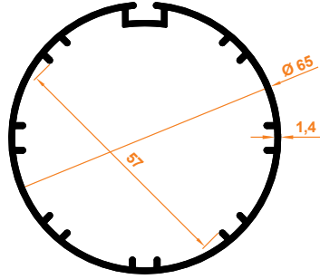
Zebra Perde 65'lik Motor Boru Zebra Blind Ø65 Motor Tube
