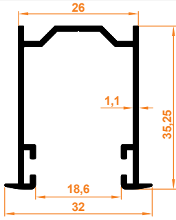
Kulaklı Kutusuz Dikme Profil Lugged Boxless Mullion Profile
