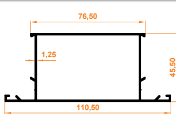
Aldoks (Geniş) Orta Kayıt Profili Aldoks (Wide) Mid Entry Profile
