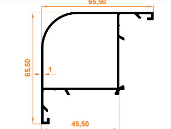
Aldoks Oval Köşe Dönüş Profili Aldoks Oval Corner Profile
