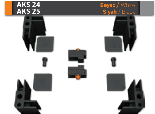
Süper Seri Büyük Köşeden Gergi Aksesuar Seti Super Serie Big Corner Tensioner Accessory Set
