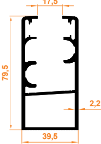
Büyük Düz Kasa Profili Big Flat Case Profile
