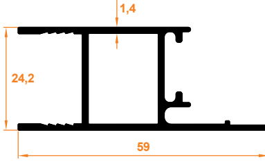
İspanyolet Dikme Profil Espagnolette Mullion Profile
