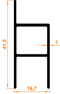
Nobel İçten/Dıştan Montajlı Kasa Profil Nobel Inside/Outside Mounted Case Profile
