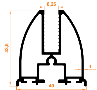
Firtına Baza Profil Firtına Base Profile
