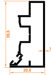
Yan Dikme Profili Side Column Profile
