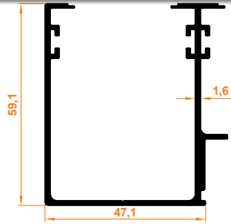
Yan U Profil Seitliches U-Profil
