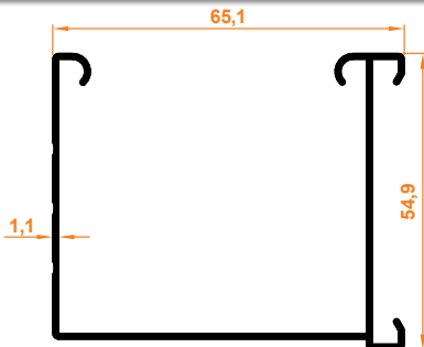
Ahşap Jaluzi Perde Kasa Profil Oberschienenprofil für Jalousien
