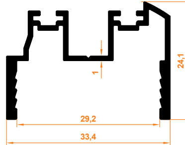
Açılı Dönüş Menteşe Profili Rücklaufscharnierprofil
