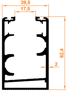
Düz Kasa Üstten Fitilli Profil Flachprofil mit Dichtung Oben
