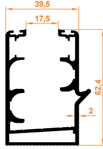
Oluklu Kasa Üstten Fitilli Profil Rinnenprofil mit Dichtung Oben
