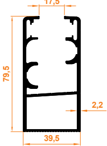
Büyük Düz Kasa Profili Großes Flachprofil
