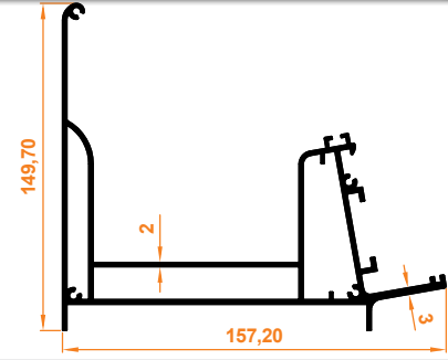
Oluk Profili Rinnenprofil
