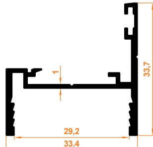
Sabit Cam Kilit Profil Schließprofil (Tij) für Festglas
