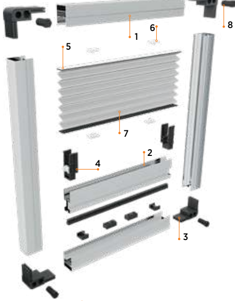
Köşeden Gergi Set İçeriği / Set-Inhalt mit Eckspann
