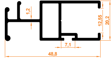
Platin Kanat Profil Platin Serie Flügelprofil
