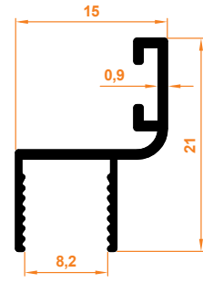
Küçük h Fitol Dichtungprofil h (klein)
