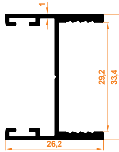
Düz Kapak Profili Isolierglas-Flachabdeckprofil
