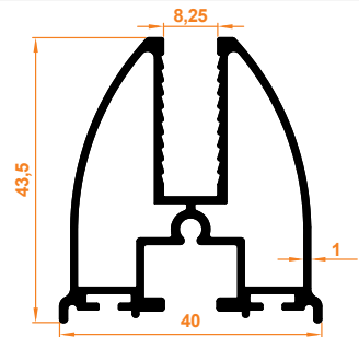
Fırtına Baza Profil Fırtına Bodenprofil
