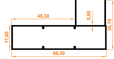
Süper Büyük Kasa Profili Super Großserie Rahmenprofil
