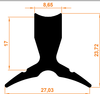
Y Bağlantı Profil Y-Connector Profile
