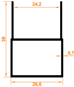
Junior Kasa Profil Junior Rahmenprofil
