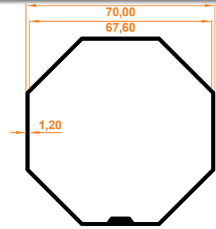
Sac Tambur Borusu Blech-Trommelrohr
