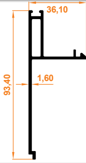
Kasa Kapatma Profili Abdeckungsprofil
