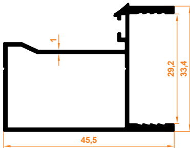
90° Dönüş Profil 90°-Drehungsprofil
