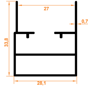
Star Kasa Profil Star Rahmenprofil
