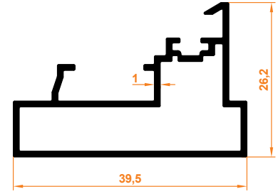
Açılır Dikme Profil Rahmenprofil Öffnend
