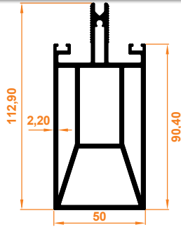
Destekli Orta Kayıt Profili Aluminium Sparren (verstärkt)
