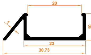
Süper Eşiksiz Kasa Profil Super-Türrahmenprofil ohne Schwelle
