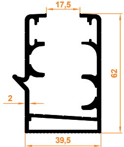
Oluklu Kasa Profili Rinnenprofil
