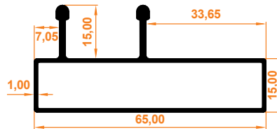
Platin Geniş Çiftli Kasa Profil Platin Breites Doppel-Rahmenprofil
