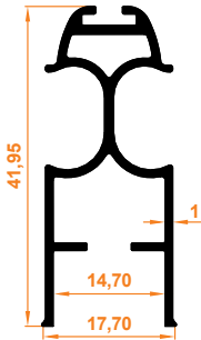
Nobel Kanat Profili
