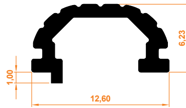
Yaylı Portray Profil Portray-Profil mit Feder
