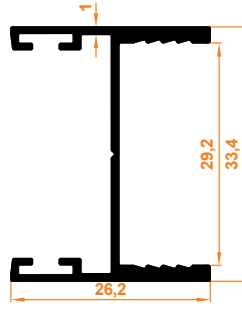
Düz Kapak Profil Isolierglas-Flachabdeckprofil
