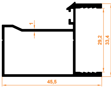
90° Dönüş Profili 90°-Drehungsprofil
