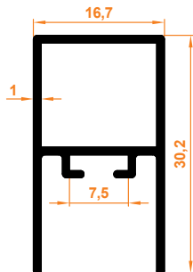
Nobel Mıknatıs Yuvalı Kasa Profili
