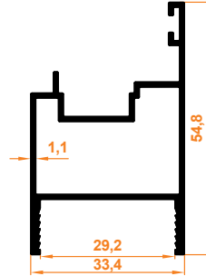
Sabit Cam İspanyolet Profil Drehstangengriff Profil für Festglas
