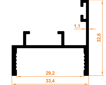
Sabit Cam İspanyolet Karşılık Profil Gegenstück Profil 8 mm Drehstangengriff für Festglas
