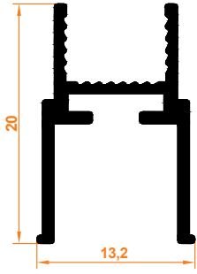
Orta H Fitol Dichtungprofil H (mitte)
