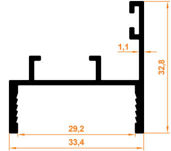
Sabit Cam İspanyolet Karşılık Profil Gegenstück Profil 8 mm Drehstangengriff für Festglas
