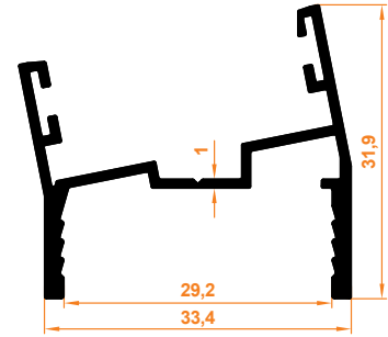
11° Dönüş Profil 11°-Drehungsprofil
