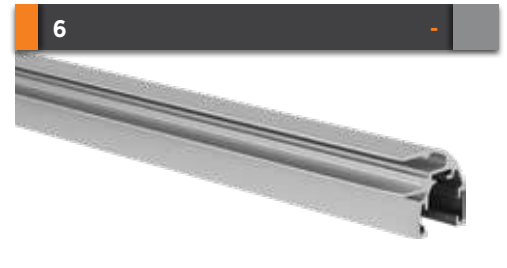
Küçük h Fitil Dichtungsprofil h (klein) Paket İçi Adet Stück im Paket 20 Gramajı Gewicht 0,116 kg/m
