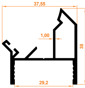
45° Dönüş Profil 45°-Drehungsprofil
