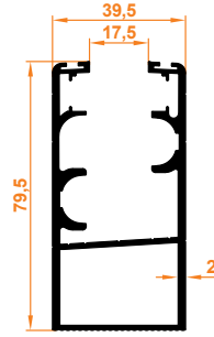
Üstten Fitilli Büyük Düz Kasa Großes Flachprofil mit Dichtung Oben
