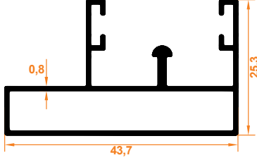
Aykim Kasa Profil Aykim Rahmenprofil
