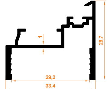
Sabit Cam Kilit Karşılığı Profil Schließprofil Gegenstück (Tij) für Festglas
