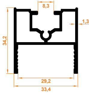
Baza Profil Isolierglas-Bodenprofil
