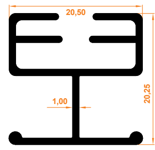
20'lik T Profil 20' er T-Profil
