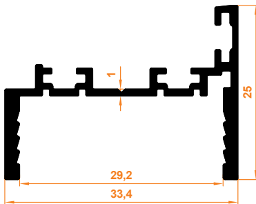
Sabit Cam Menteşe Profil Scharnierprofil für Festglas
