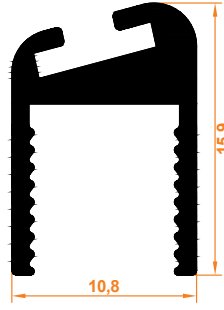
Küçük D Fitol Dichtungprofil D (klein)
