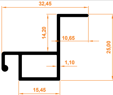
İçten Montajlı Sabit Sineklik Kasa Profil
