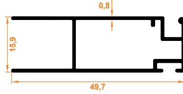
Aykim Hareketli Profil Aykim Flügelprofil
