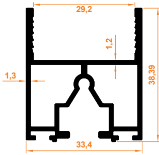
Fitilli Baza Profili Dichtungsbodenprofil
