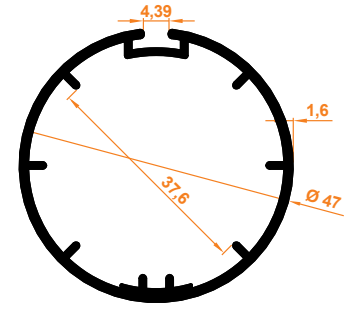
Zebra Perde 47'lik Motor Boru Zebra-Rollo Ø47 Motorrohr
