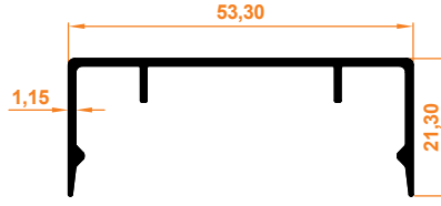
Cam Çita Kapak Profili Glasleisten Abdeckungsprofil
