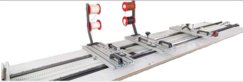
İp Ayar Boylama Tezgahı Plissee-Schnureinstellungsmaschine
