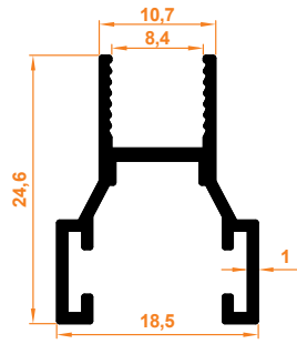
Büyük H Fitol Dichtungprofil H (groß)
