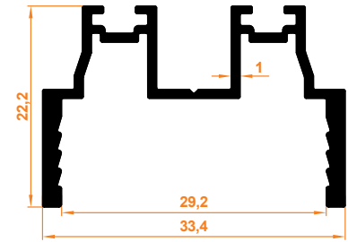
Düz Kapak Menteşe Profili Abdeckung Isolierglas-Scharnierprofil
