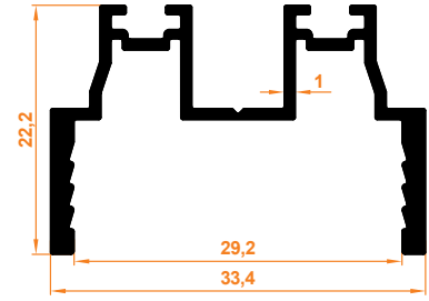
Düz Kapak Menteşe Profil Abdeckung Isolierglas-Scharnierprofil
