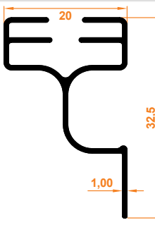
Etekli 20'lik T Profil 20' er T-Profil mit Blende
