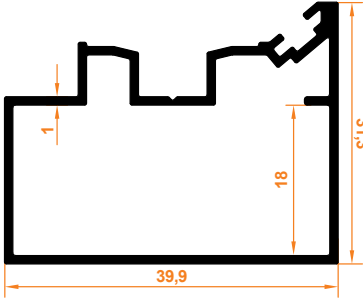
Geniş Yan Dikme Rahmenprofil Isolierglas Breit
