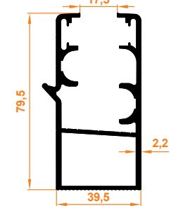
Oluklu Büyük Kasa Profili Großes Rinnenprofil
