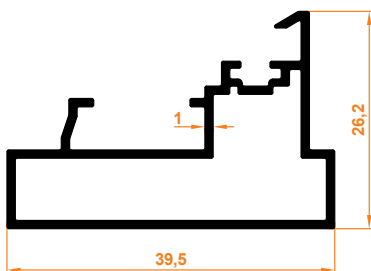
Açılır Dikme Profili Rahmenprofil Öffnend
