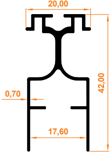
Süper Seri Kanat Profili Super Flügelprofil
