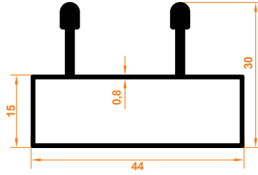
Platin Çiftli Kasa Profil Platin Serie Rahmenprofil – zweiflügelig
