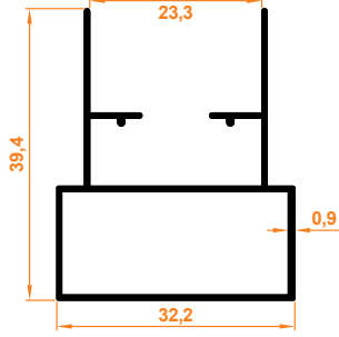
Gold Kasa Profil Gold Rahmenprofil
