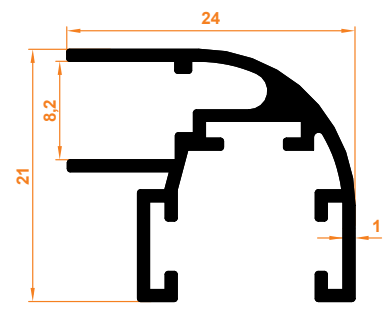
Köşe Dönüş Fitol Dichtungprofil Eck-Rücklauf
