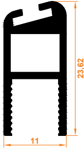
Büyük D Fitol Dichtungprofil D (groß)
