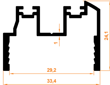
Açılı Dönüş Menteşe Profil Rücklaufscharnierprofil
