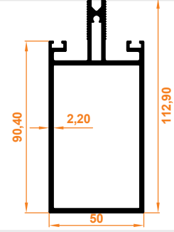
Orta Kayıt Profili Aluminium Sparren
