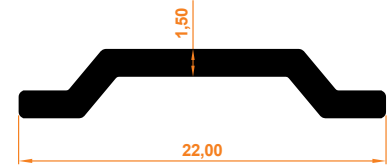
Tij Profil Getriebeprofil
