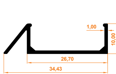
Junior Eşiksiz Kasa Profil Junior Bodenprofil - mit niedriger Schwelle
