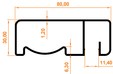
80x30 Yandan Kanallı 80x30 Side Slot
