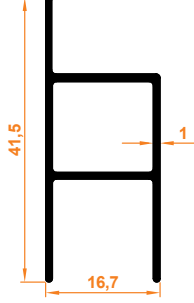
Nobel İçten/Dıştan Montajlı Kasa Profil
