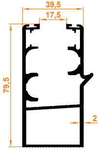
Üstten Fitilli Büyük Oluklu Kasa Großes Rinnenprofil mit Dichtung Oben
