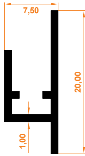
Yaylı Yapışkan Profil Klebspfil mit Spannfeder
