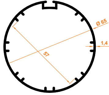
Zebra Perde 65'lik Motor Boru Zebra-Rollo Ø65 Motorrohr
