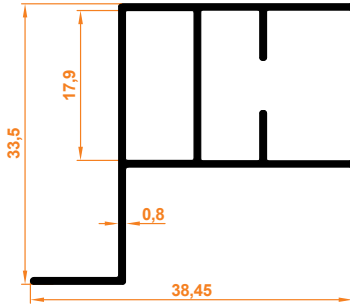
Slim Seri İçten Montajlı Kasa Profil
