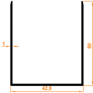
U Kapatma Profil U-Abschlussprofil
