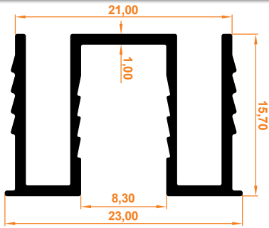
8 mm Cam Adaptörü Einscheiben-Glas-Adapter
