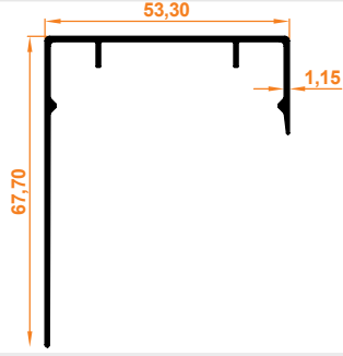
Sonlandırıcı Cam Çita Kapak Profili Endkappe Glasleiste Abdeckprofil
