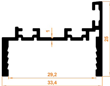
Sabit Cam Menteşe Profili Scharnierprofil für Festglas
