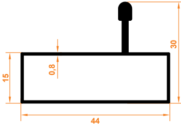
Platin Tekli Kasa Profil Platin Serie Rahmenprofil – einflügelig
