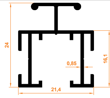
Çiftli Orta Profil Mittleres Doppelprofil
