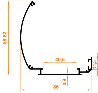
Kapalı Kasa Geniş Profil Breites Geschlossenes Kastenprofil
