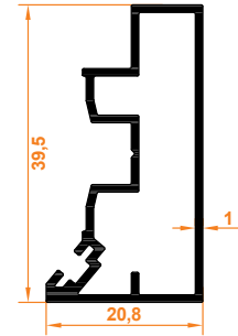
Yan Dikme Profili Rahmenprofil Isolierglas
