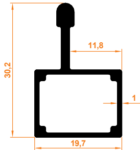
Platin Tekli Dar Kasa Profil Platin Serie Rahmenprofil – einflügelig, schmal
