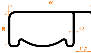
60x25 Yandan Kanallı 60x25 Side Slot
