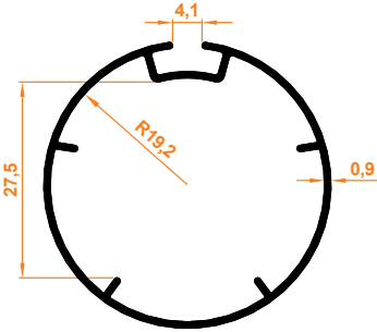
Zebra Perde Borusu Zebra Blind Tube
