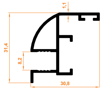
8 mm İspanyolet Profil Karşılığı 8 mm Espagnolette Combination Profile
