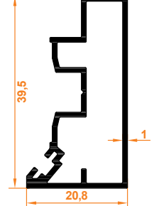
Yan Dikme Profili Side Column Profile
