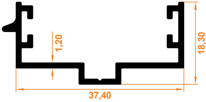
Birleştirme Karşılık Profil Combination Provisions Profile
