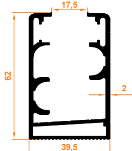
Düz Kasa Profili Flat Case Profile
