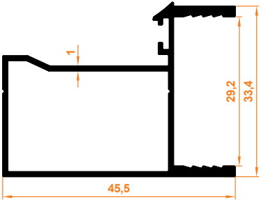
90° Dönüş Profili 90° Return Profile
