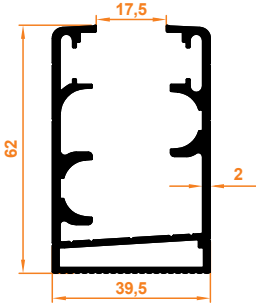
Düz Kasa Profil Flat Case Profile
