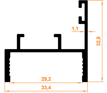
Sabit Cam İspanyolet Karşılık Profil Fixed Glass Espagnolette Handle Provision Profile
