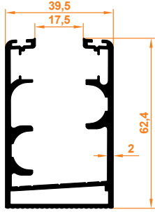
Düz Kasa Üstten Fitilli Profil Flat Case Top Wicked Profile
