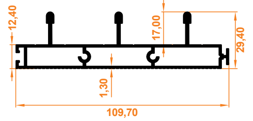
Üçlü Eşikli Alt Kasa Profil Triple Threshold Lower Case Profile
