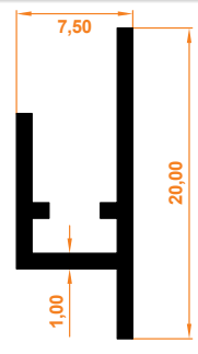
Yaylı Yapışkan Profil Spring Adhesive Profile
