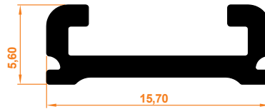
Portray Yapışkan Profil Adhesive Profile
