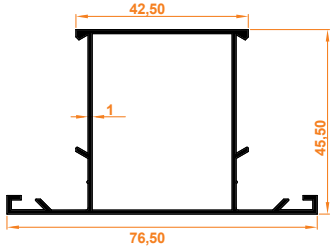
Aldoks (Orta) Kayıt Profili Aldoks (Mid) Entry Profile
