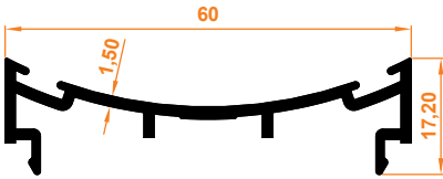
C60 Çarpma Kapı Adaptörü - Dişi C60 Crash Door Adapter - Female
