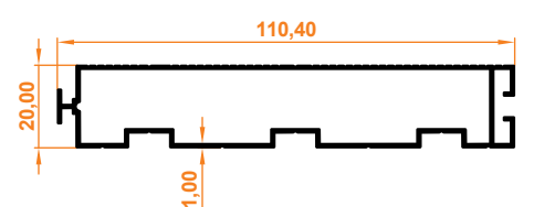
Üçlü Yan Kasa Profil Triple Side Case Profile
