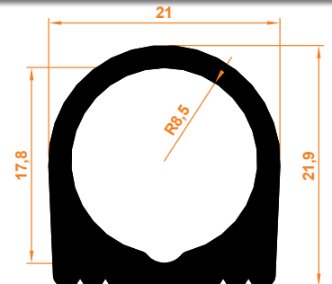
Boru Tutamak Profil Tube Grip Profile
