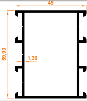
C60 Kasa Orta Kayıt Profili C60 Case Mid Entry Profile
