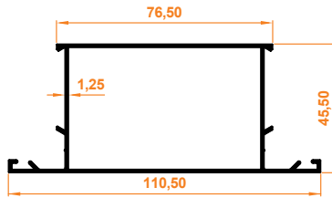
Aldoks (Geniş) Orta Kayıt Profili Aldoks (Wide) Mid Entry Profile
