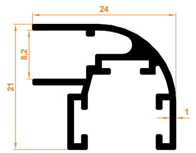
Köşe Dönüş Fitil Corner Return Wick
