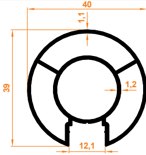
40x1,1 mm Tek Kanallı Çiftli Dikme 40x1,1 mm Single Channel Double Column
