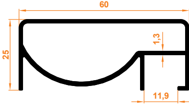
60x25 mm Üst Küpeşte Yandan Kanallı 60x25 mm Upper Handrail with Side Channel
