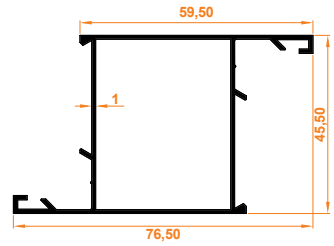
Aldoks (Orta) Kanat Profili Aldoks (Mid) Wing Profile
