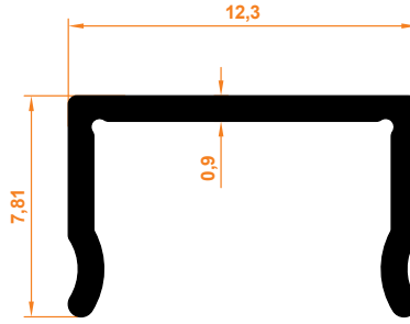
Kare Çıta Square Slat
