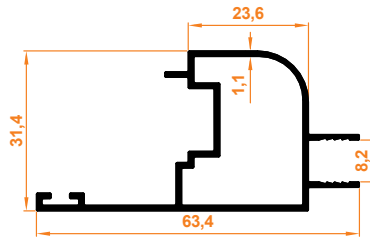
8 mm İspanyolet Profil 8 mm Espagnolette Profile
