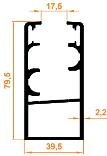
Büyük Düz Kasa Profil Big Flat Case Profile
