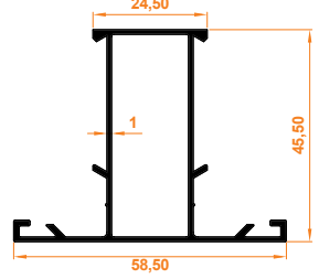
Aldoks (Dar) Orta Kayıt Profili Aldoks (Tight) Mid Entry Profile
