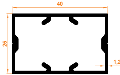
40x25 Dikme 40x25 Column
