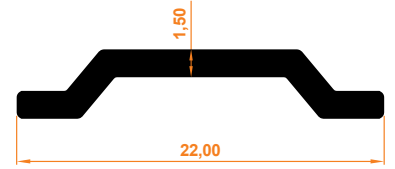
Tij Profil Espagnolette Profile
