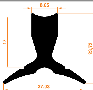
Y Bağlantı Profil Y-Connector Profile
