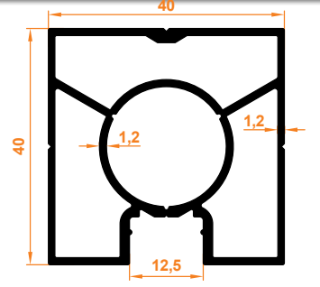
40x40 Tek Kanallı Dikme 40x40 Single Channel Column
