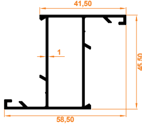
Aldoks (Dar) Kanat Profili Aldoks (Tight) Wing Profile
