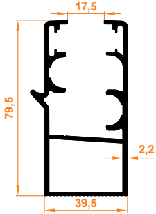
Oluklu Büyük Kasa Profil Corrugated Big Case Profile
