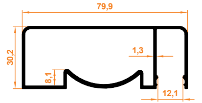
80x30 Yandan Kanallı 80x30 Side Channel
