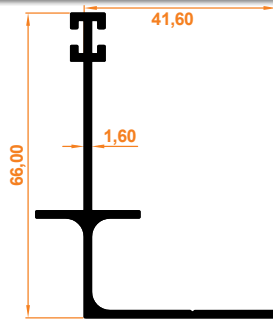
Açılımsız Çift Fıtil Yan Ray L Kasa Profil Double Weatherstrips Without Opening Side L Case Profile
