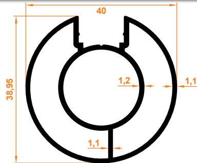
40x1,1 mm Tek Kanallı Tekli Dikme 40x1,1 mm Single Channel Single Column
