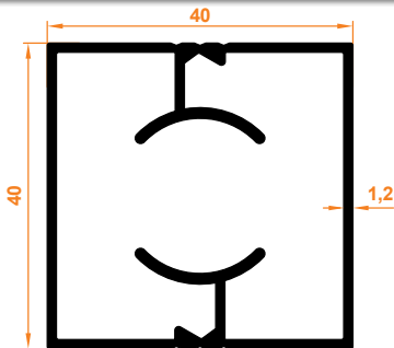
40x40 Kanalsız Dikme 40x40 Non Channel Column
