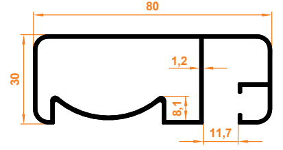
80x30 Yandan Kanallı 80x30 Side Channel
