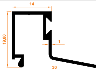
Aldoks Isıcam Çita Aldoks Double Glazing Stave
