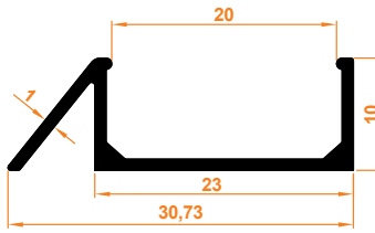
Süper Eşiksiz Kasa Profil Super without Threshold Case Profile
