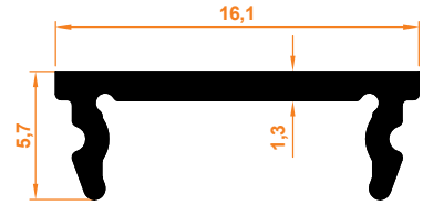
Takviyesiz Cam Tutucu Çıta Profil Non-Reinforced Glass Holder Lath Profile
