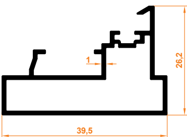
Açılır Dikme Profili PopUp Column Profile
