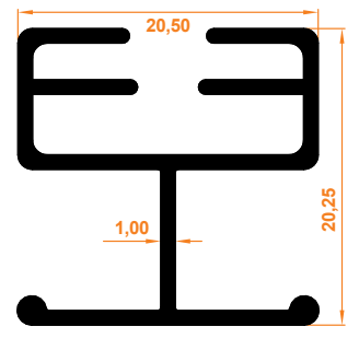
20'lik T Profil 20 T Profile
