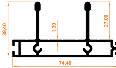
İkili Üst Kasa Profil Double Upper Case Profile
