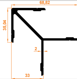
Aldoks (Orta) Köşe Takoğu Aldoks (Mid) Corner Wedge
