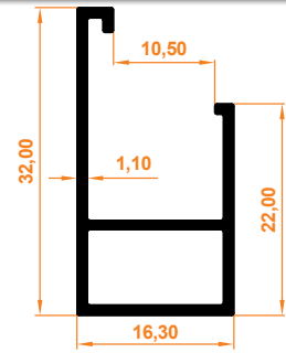
8-10 mm Cam Altı Profil 8-10 mm Glass Bottom
