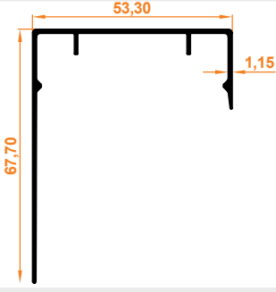
Sonlandırıcı Cam Çita Kapak Profili End Cap Glass Strip Cover Profile
