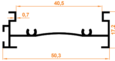
Zebra Açık Kasa Open Cassette for Zebra Blinds
