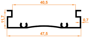
Stor Perde Kasa Tırnaksız Toothless Headbox for Roller Blinds
