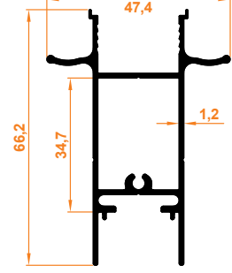
İspanyolet Çekme Kol Profili Espagnolette Pull Handle Profile
