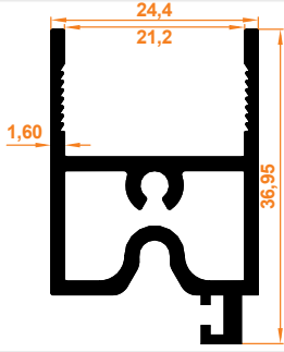
Sabit Panel Açılır Alt Baza Profil Fixed Panel Pop-up Base Profile
