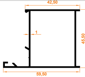
Aldoks (Orta) Kasa Profili Aldoks (Mid) Frame Profile
