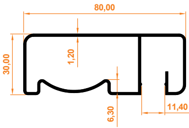
80x30 Yandan Kanallı 80x30 Side Slot
