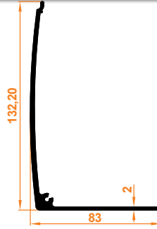
Üst Kasa Kapak Profili Upper Case Cover Profile
