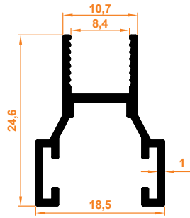
Büyük H Fitil Big H Wick
