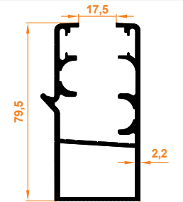
Oluklu Büyük Kasa Profili Corrugated Big Case Profile
