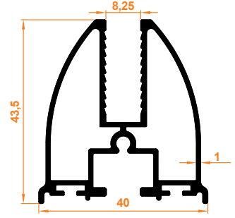
Fırtına Baza Profil Firtina Base Profile
