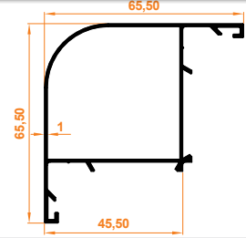
Aldoks Oval Köşe Dönüş Profili Aldoks Oval Corner Profile
