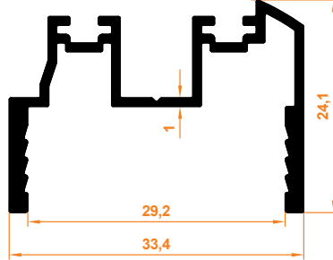
Açılı Dönüş Menteşe Profili PopUp Return Hinge Profile
