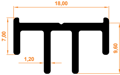
İspanyolet Karşılık Profili Espagnolette Provision Profile
