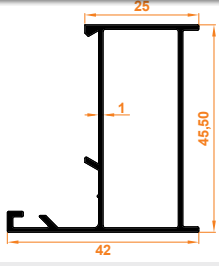
Aldoks (Dar) Kasa Profili Aldoks (Tight) Frame Profile
