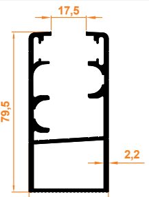
Büyük Düz Kasa Profili Big Flat Case Profile
