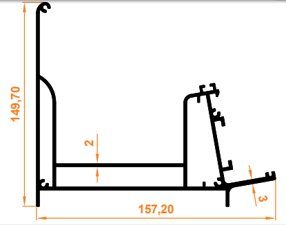
Oluk Profili Groove Profile
