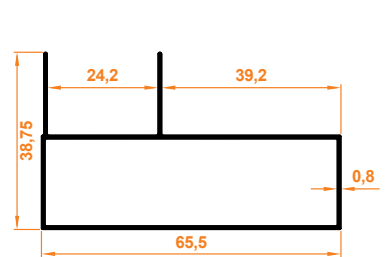
Junior Büyük Kasa Profili Junior Big Case Profile
