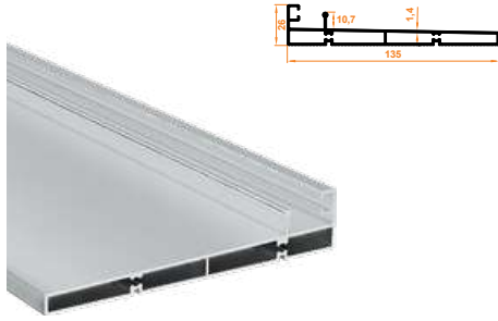
170 Alt Kasa Profil Bottom Frame Profile
