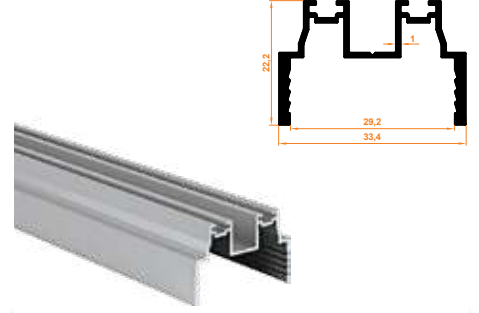
802 Düz Kapak Menteşe Profil Flat Cover Hinge Profile
