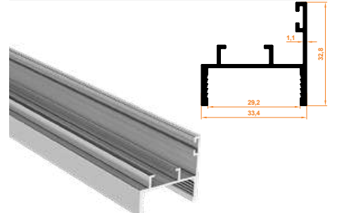
825 Sabit Cam İspanolet Karşılık Profil Fixed Glass Espagnolette Handle Provision Profile
