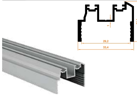
807 Açılı Dönüş Menteşe Profil PopUp Return Hinge Profile
