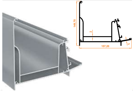
422 Oluk Profili Groove Profile
