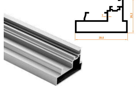
822 Açılır Dikme Profil PopUp Column Profile
