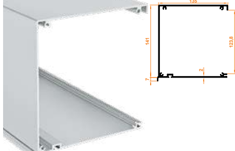
179 Üst Kasa Profil Top Frame Profile
