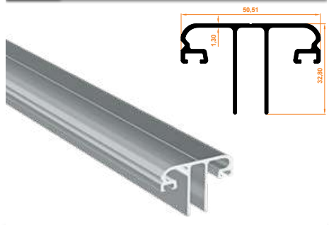
429 Cam Çitası Profili Glass Strip Profile
