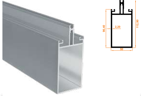
419 Orta Kayıt Profili Center Mullion Profile
