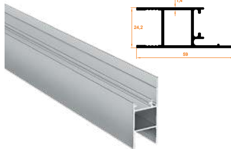
174 İspanyolet Dikme Profil Espagnolette Mullion Profile
