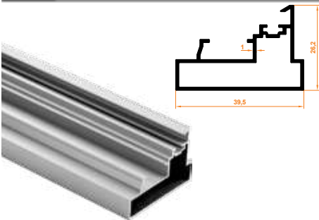
822 Açılır Dikme Profil Pop-up Column Profile
