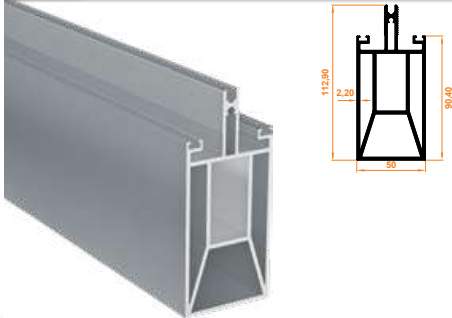
423 Mukavemetli Orta Kayıt Profili Reinforced Center Mullion Profile
