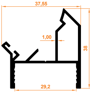
45° Dönüş Profil 45° Return Profile
