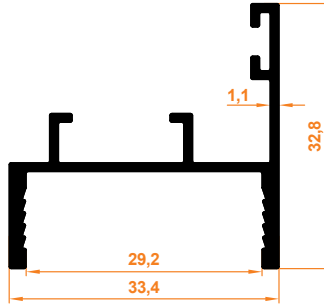
Sabit Cam İspanyolet Karşılık Profil Fixed Glass Espagnolette Handle Provision Profile
