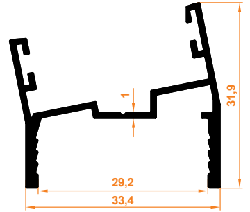
11° Dönüş Profil 11° Return Profile
