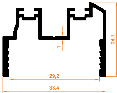
Açılı Dönüş Menteşe Profil PopUp Return Hinge Profile
