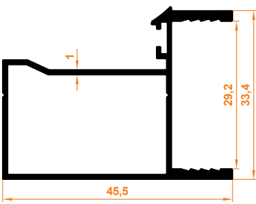
90° Dönüş Profil 90° Return Profile
