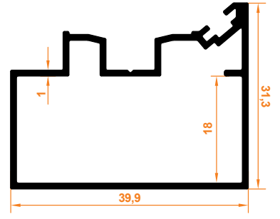
Geniş Yan Dikme Wide Side Column
