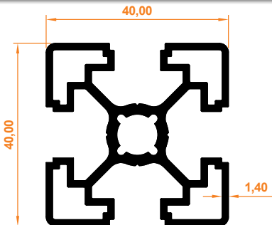
40x40 Sigma Profil 40x40 Sigma Profile
