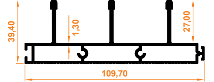
Üçlü Üst Kasa Profil Triple Upper Case Profile
