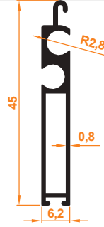
39x55 Alt Parça Kilitli Profil 39x55 Bottom Locking Profile
