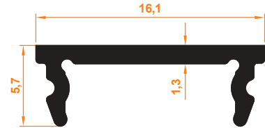
Takviyesiz Cam Tutucu Çıta Profil Non-Reinforced Glass Holder Lath Profile
