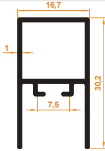
Nobel Mıknatıs Yuvalı Kasa Profili Nobel Magnet-Channel Frame Profile
