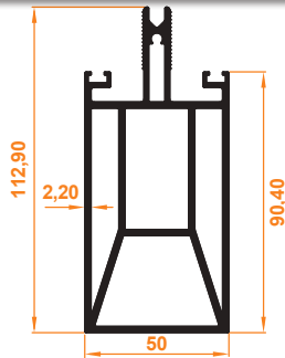
Mukavemetli Orta Kayıt Profili Reinforced Center Mullion Profile
