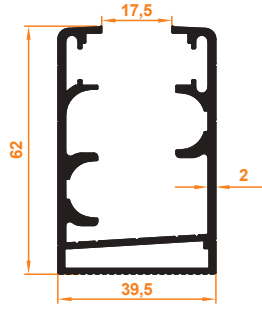
Düz Kasa Profil Flat Case Profile
