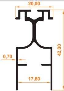
Süper Seri Kanat Profili Super Wing Profile
