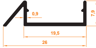
Slim Eşiksiz Profil
