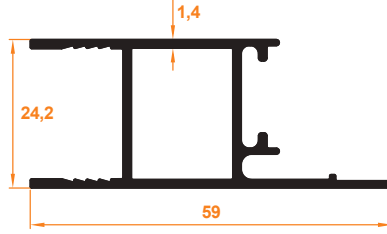
İspanyolet Dikme Profil Espagnolette Mullion Profile
