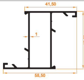
Aldoks (Dar) Kanat Profili Aldoks (Tight) Wing Profile
