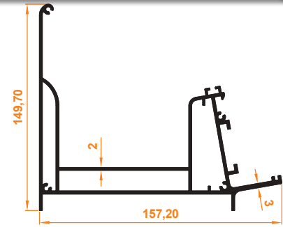
Oluk Profili Groove Profile
