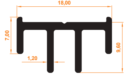
İspanyolet Karşılık Profili Espagnolette Provision Profile
