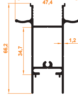
İspanyolet Çekme Kol Profili Espagnolette Pull Handle Profile
