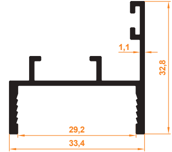
Sabit Cam İspanyolet Karşılık Profil Fixed Glass Espagnolette Handle Provision Profile
