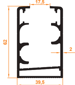
Düz Kasa Profili Flat Case Profile
