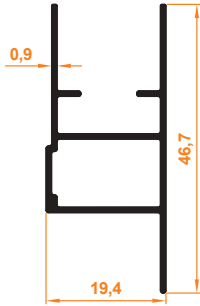
Nova İçten/Dıştan Montajlı Kasa Profil Nova Inside/Outside Mounted Case Profile
