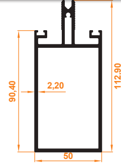
Orta Kayıt Profili Center Mullion Profile
