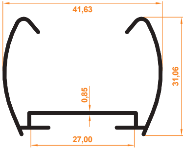
Aura Üst Kasa Profili Aura Upper Case Profile
