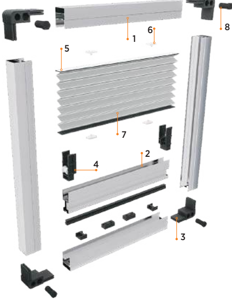
Köşeden Gergi Set İçeriği / Corner Tensioner Set Contents
