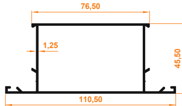
Aldoks (Geniş) Orta Kayıt Profili Aldoks (Wide) Mid Entry Profile
