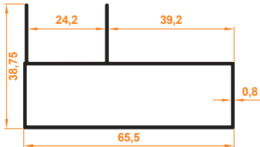
Junior Büyük Kasa Profili Junior Big Case Profile
