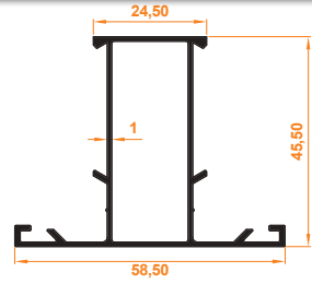
Aldoks (Dar) Orta Kayıt Profili Aldoks (Tight) Mid Entry Profile
