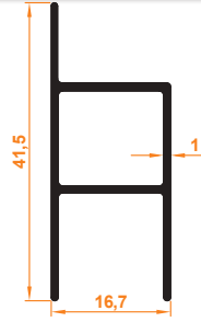
Nobel İçten/Dıştan Montajlı Kasa Profili Nobel Inside/Outside Mounted Case Profile
