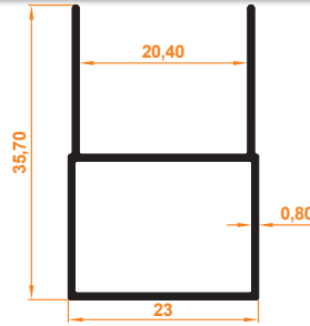
Süper Seri Kasa Profili Super Case Profile
