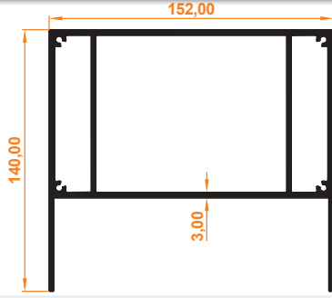
Taşıyıcı Profili Carrier Profile
