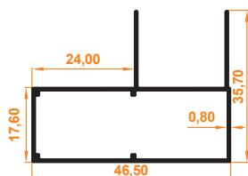
Süper Orta Kasa Profili Super Middle Case Profile
