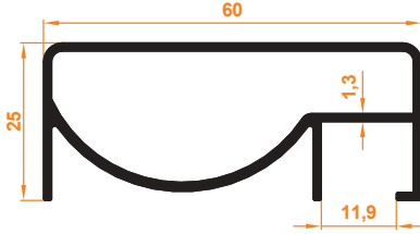
60x25 mm Üst Küpeşte Yandan Kanallı 60x25 mm Upper Handrail with Side Channel
