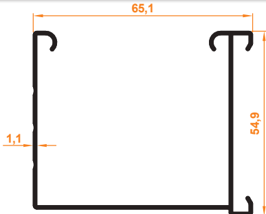
Ahşap Jaluzi Perde Kasa Profili Venetian Blind Headrail Profile
