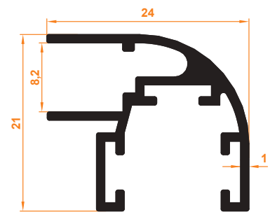
Köşe Dönüş Fitil Corner Return Wick
