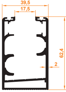
Düz Kasa Üstten Fitilli Profil Flat Case Top Wicked Profile
