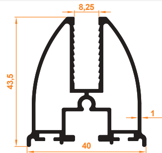
Fırtına Baza Profil Fırtına Base Profile
