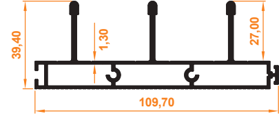
İkili Üçlü Kasa Profil Triple Upper Case Profile
