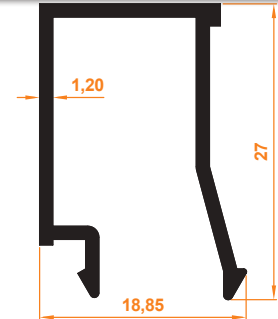
C60 Isıcam Çıta Profili C60 Insulating Glass Stave Profile
