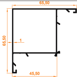
Aldoks Köşe Dönüş Profili Aldoks Corner Profile
