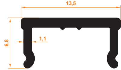
80x30 Yandan Kanallı Çıtası 80x30 Side Slot Rail
