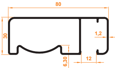
80x30 Yandan Kanallı 80x30 Side Slot
