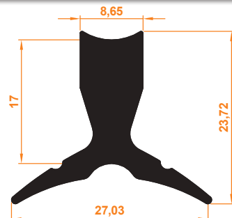
Y Bağlantı Profil Y-Connector Profile
