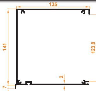
Üst Kasa Profil Top Frame Profile
