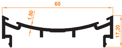
C60 Çarpma Kapı Adaptörü - Dişi C60 Crash Door Adapter - Female
