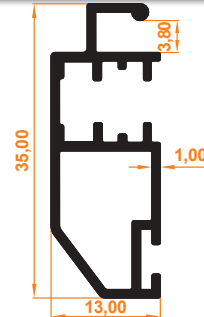
13x35 Dıştan Montajlı Sineklik Profil 13x35 Externally Mounted Fly Screen Profile
