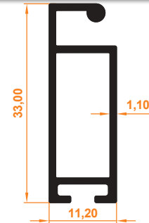
Fitilli Dıştan Montajlı Sineklik Profil External-Mount Fly Screen Profile with Wick
