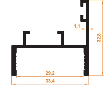
Sabit Cam İspanyolet Karşılık Profil Fixed Glass Espagnolette Handle Provision Profile
