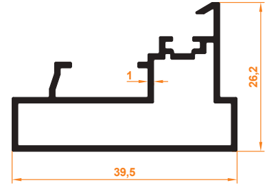
Açılır Dikme Profil PopUp Column Profile
