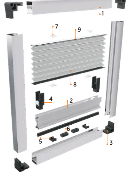
İçten Gergi Set İçeriği / Internal Tensioner Set Contents
