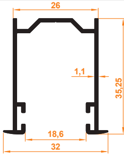
Kulaklı Kutusuz Dikme Profil Lugged Boxless Mullion Profile
