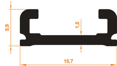
Portray Yapışkan Profil Adhesive Profile
