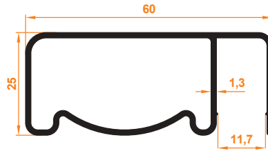
60x25 Yandan Kanallı 60x25 Side Slot
