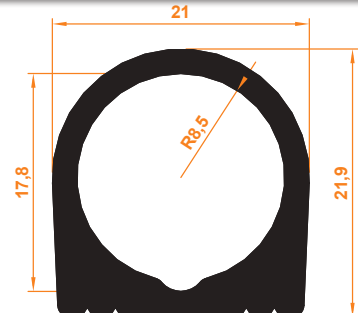
Boru Tutamak Profil Tube Grip Profile
