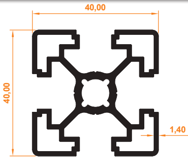
40x40 Sigma Profil 40x40 Sigma Profile
