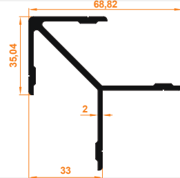
Aldoks (Orta) Köşe Takozu Aldoks (Mid) Corner Wedge
