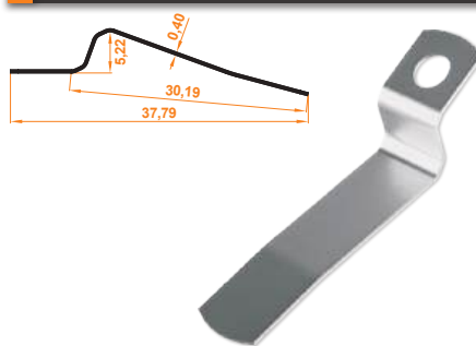
Dıştan Montajlı Metal Klips Externally Mounted Metal Clip
