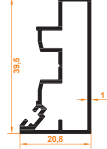
Yan Dikme Profili Side Column Profile
