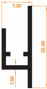
Yaylı Yapışkan Profil Spring Adhesive Profile
