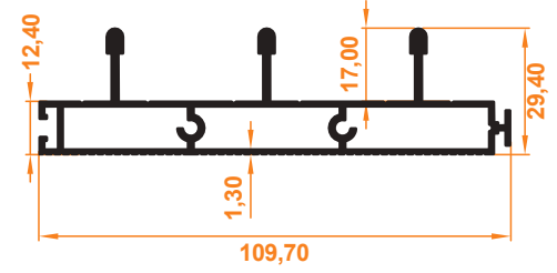
Üçlü Eşikli Alt Kasa Profil Triple Threshold Lower Case Profile
