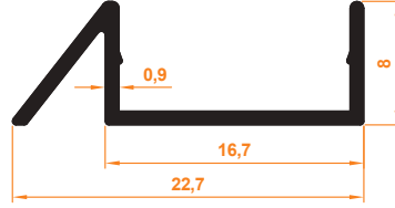
Nobel Eşiksiz Profili Nobel Profile without Threshold
