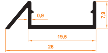
Nova Eşiksiz Profil Nova Profile without Threshold
