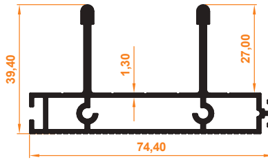
İkili Üst Kasa Profil Double Upper Case Profile
