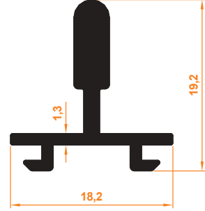
Platin Orta Birleştirme Profil Platin Center Joining Profile
