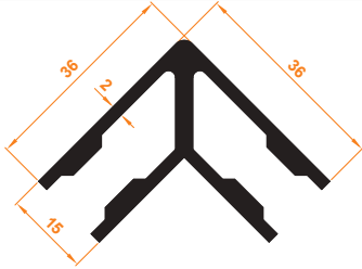
Aldoks (Dar) Köşe Takozu Aldoks (Tight) Corner Wedge
