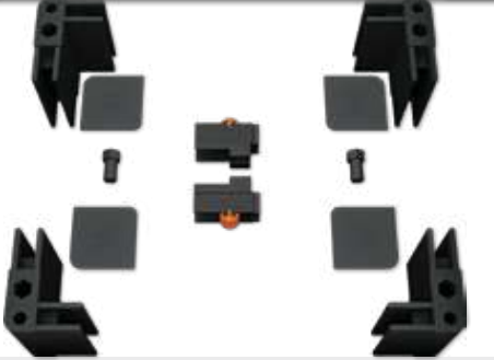
Süper Seri Orta Köşeden Gergi Aksesuar Seti Super Serie Middle Corner Tensioner Accessory Set
