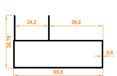
Junior Büyük Kasa Profili Junior großem Rahmenprofil
