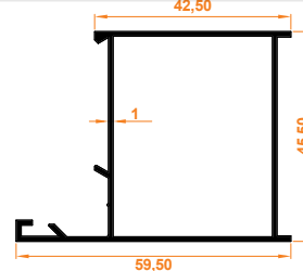
Aldoks (Orta) Kasa Profili Aldoks (Medium) Frame Profile
