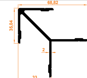
Aldoks (Orta) Köşe Takozu Aldoks (Medium) Corner Wedge
