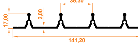
Dörtlü Eşiksiz Alt Kasa Profil Quadruple Bottom Case Profile without Threshold
