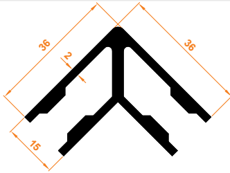
Aldoks (Dar) Köşe Takozu Aldoks (Narrow) Corner Wedge
