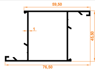
Aldoks (Orta) Kanat Profili Aldoks (Medium) Airfoil
