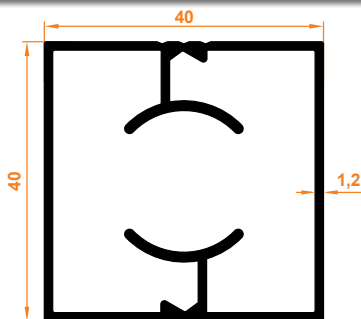
40x40 Kanalsız Dikme 40x40 Non Slot Column
