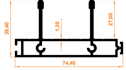
İkili Üst Kasa Profili Double Upper Case Profile
