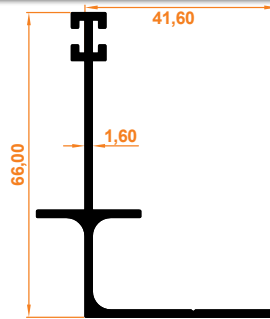
Açılımsız Çift Fıtil Yan Ray L Kasa Profil Double Weatherstrips Without Opening Side L Case Profil
