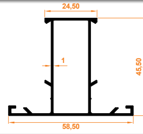
Aldoks (Dar) Orta Kayıt Profili Aldoks (Narrow) Medium Entry Profile
