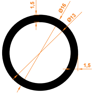
16x1,5 Boru 16x1,5 Pipe
