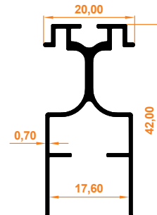
Süper Seri Kanat Profili Super Wing Profile
