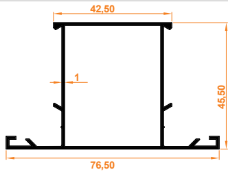
Aldoks (Orta) Orta Kayıt Profili Aldoks (Medium) Medium Entry Profile
