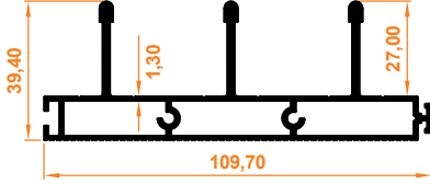
İkili Üçlü Kasa Profili Triple Upper Case Profile
