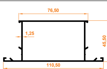
Aldoks (Geniş) Orta Kayıt Profili Aldoks (Wide) Medium Entry Profile
