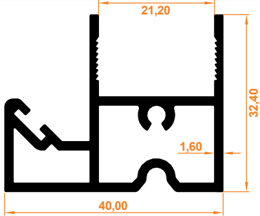
Hareketli Panel Açılır Alt Baza Profil Movable Panel Pop-up Lower Base Profile
