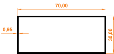
30x70 Kutu Profil 30x70 Box Profile
