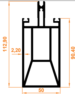
Destekli Orta Kayıt Profili Reinforced Center Mullion Profile
