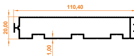
Üçlü Yan Kasa Profil Triple Side Case Profile
