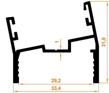
11° Dönüş Profil 11° Return Profile
