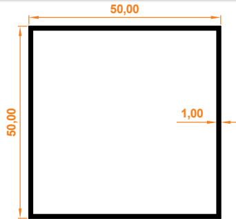
50x50 Kutu Profil 50x50 Box Profile
