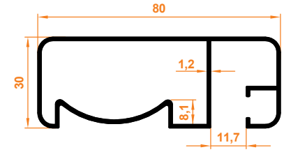
80x30 Yandan Kanallı 80x30 Side Slot
