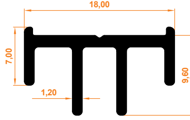
İspanyolet Karşılık Profili Espagnolette Provision Profile
