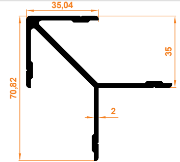
C60 Köşe Takozu C60 Corner Wedge
