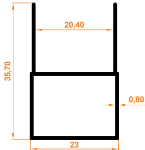
Süper Seri Profili Super Case Profile
