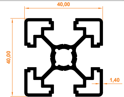
40x40 Sigma Profil 40x40 Sigma Profile
