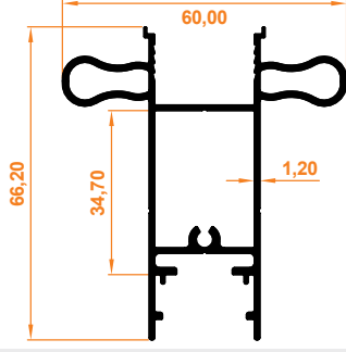
İspanyolet Çekme Kol Profili Espagnolette Pull Handle Profile
