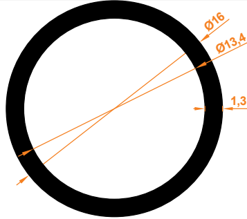
16x1,3 Boru 16x1,3 Pipe
