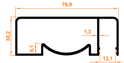
80x30 Yandan Kanallı 80x30 Side Slot
